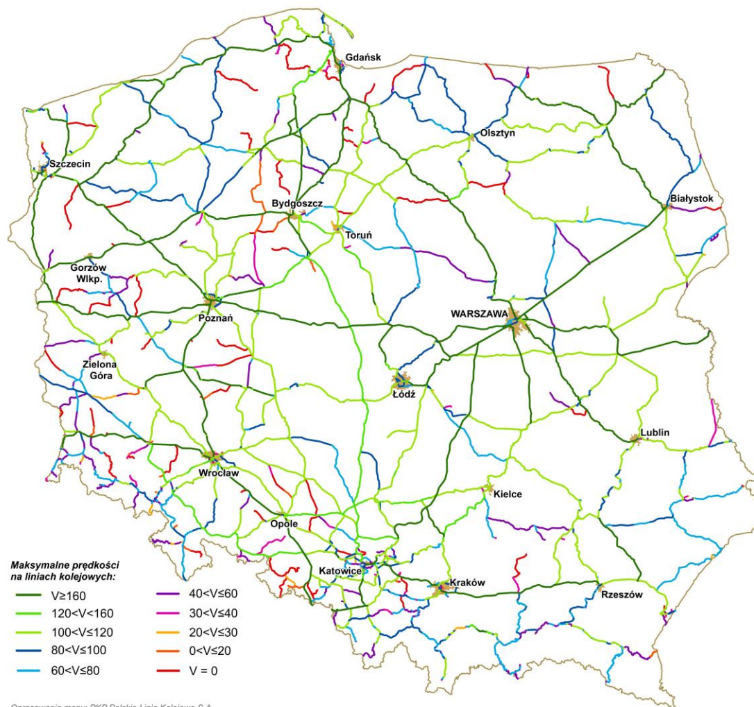
Mapa 2 – Prędkości maksymalne na liniach/odcinkach sieci kolejowej zarządzanej przez PKP PLK S.A. – prognoza na 31.12.2028 r.
