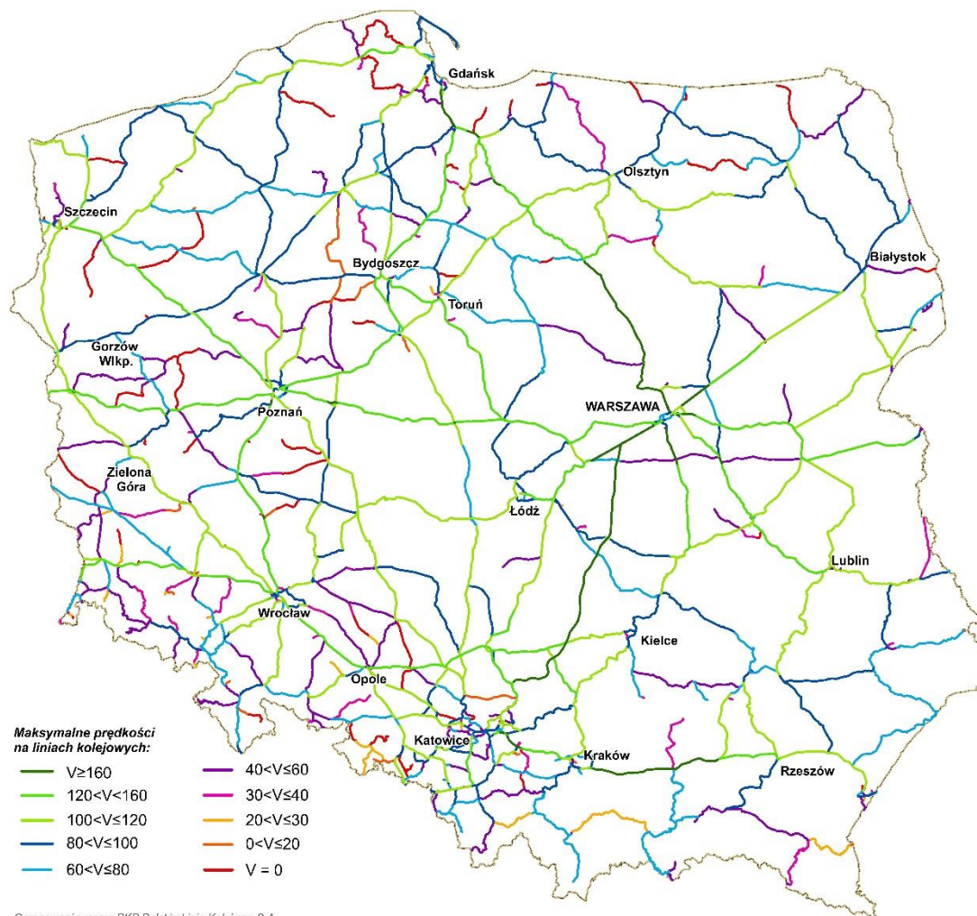
Mapa 1 – Prędkości maksymalne na liniach/odcinkach sieci kolejowej zarządzanej przez PKP PLK S.A. – stan bazowy.
