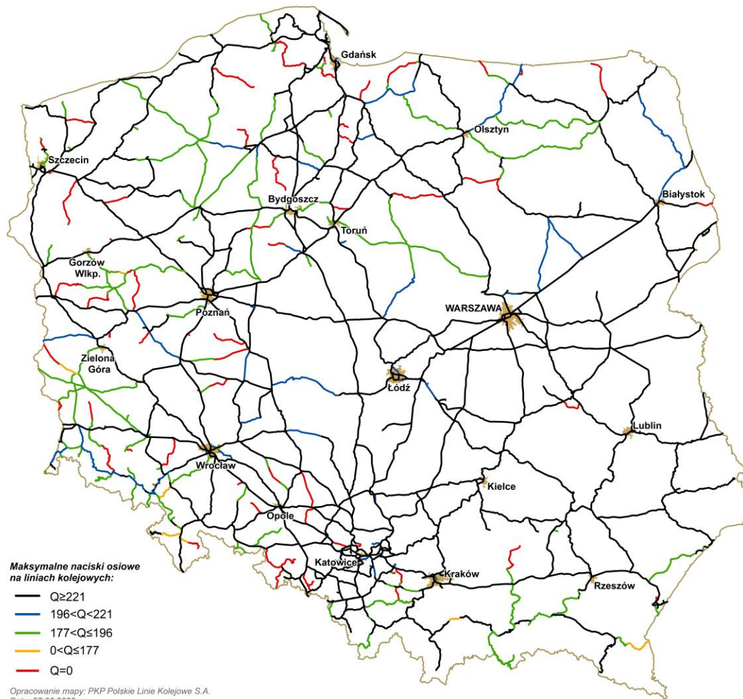
Mapa 4 – Naciski dopuszczalne osi taboru na liniach/odcinkach sieci kolejowej zarządzanej przez PKP PLK S.A. – prognoza na 31.12.2028 r.
