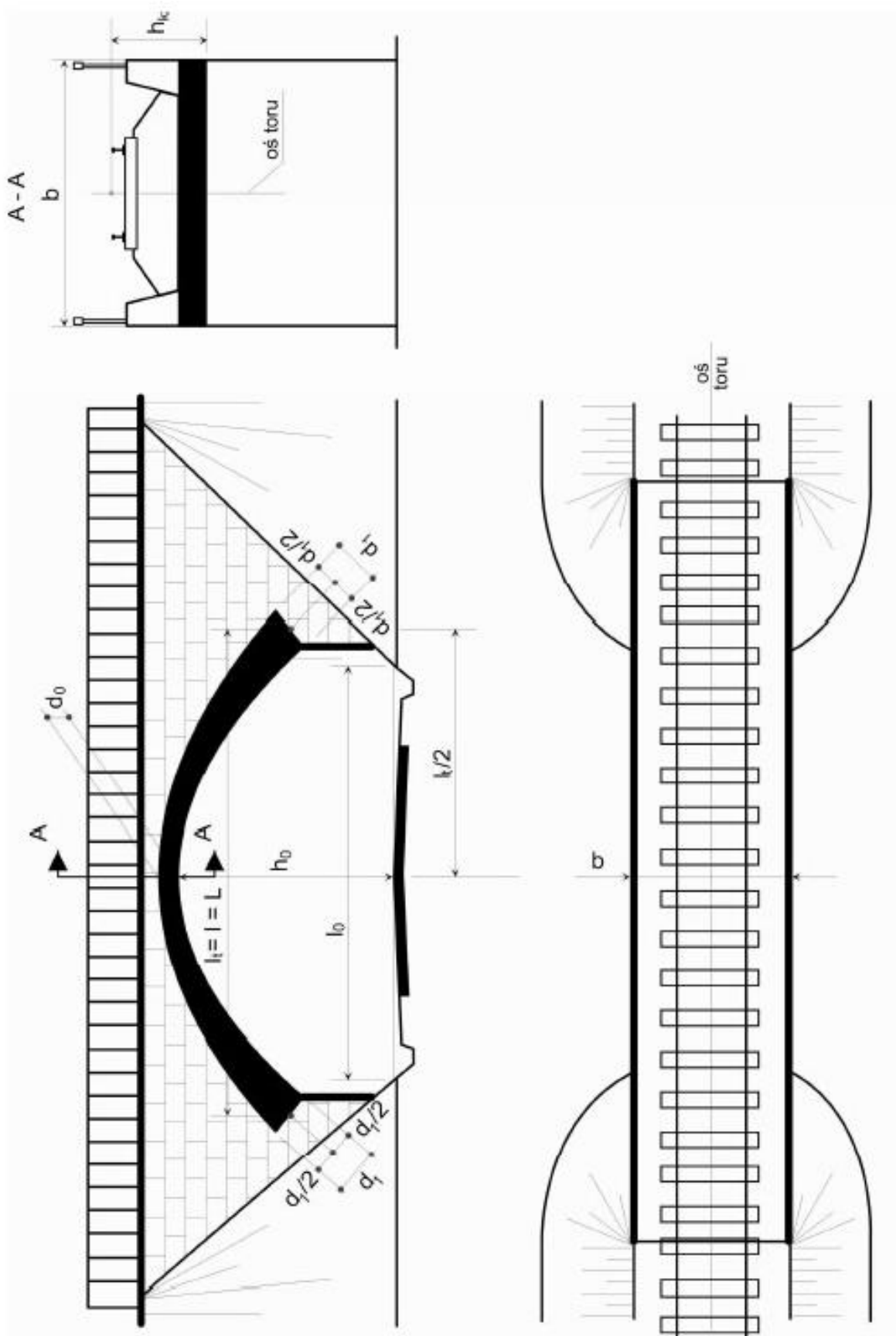
Rysunek 2.3 Rzut i przekroje poprzeczne obiektu inżynierskiego łukowego z jazdą górą
