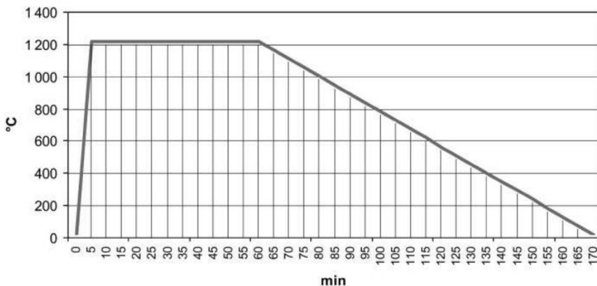
Rysunek 4. Krzywa Eureka
