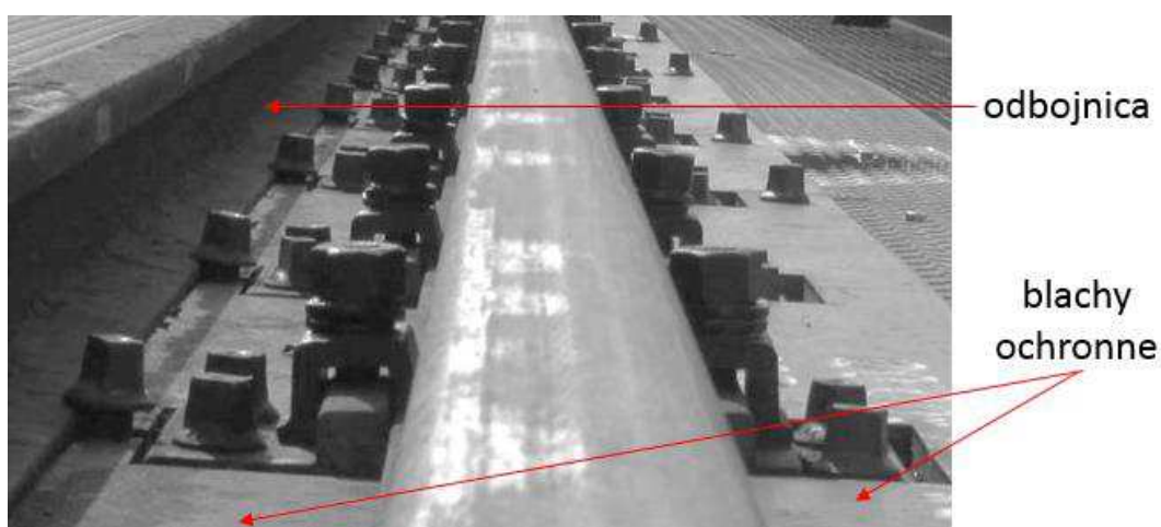
Rys. 11 Środki przeciwdziałające skutkom wykolejenia (przykładowe rozwiązanie)
