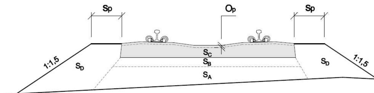
Rys. 6 Pryzma podsypki
