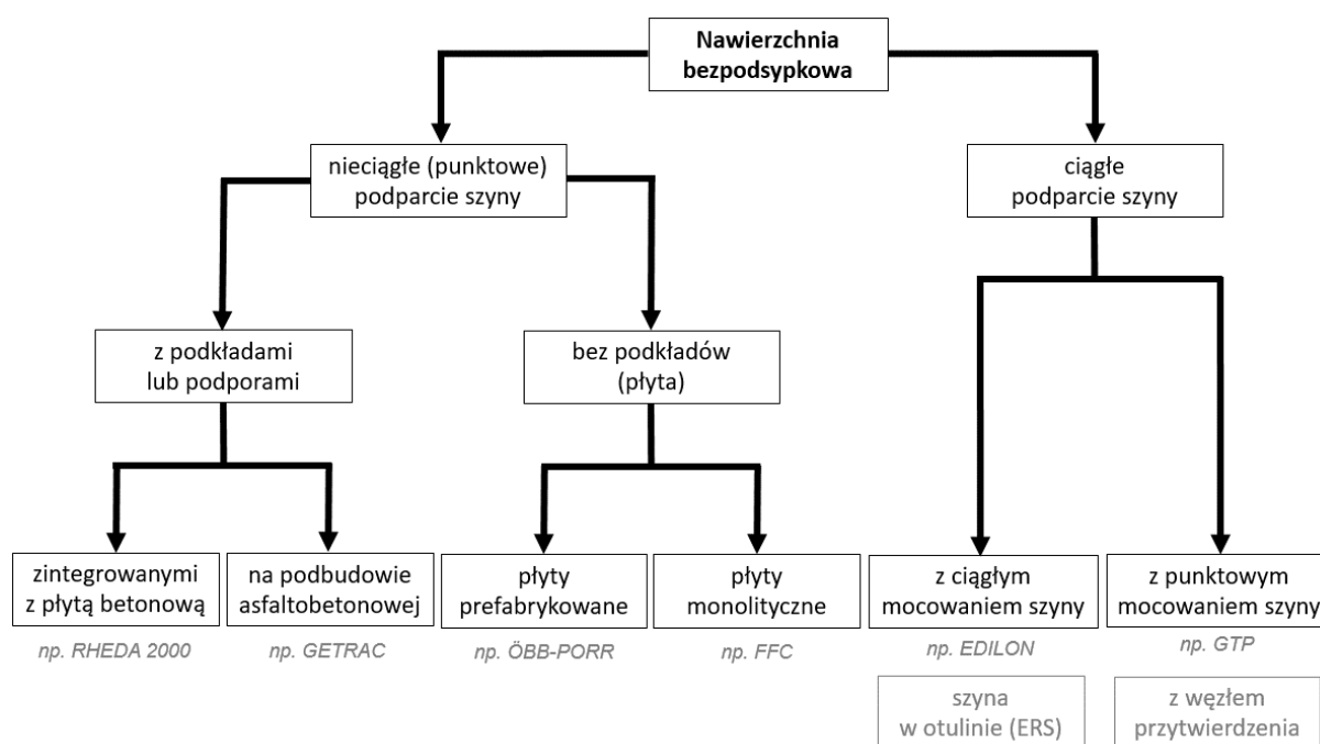
Rys. 1 Podział konstrukcji nawierzchni bezpodsypkowej
