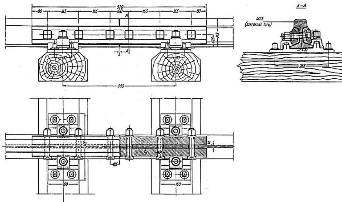
Rys.4 Złącza klasyczne „wiszące”: a) do szyn 60E1, b) do szyn 49E1
