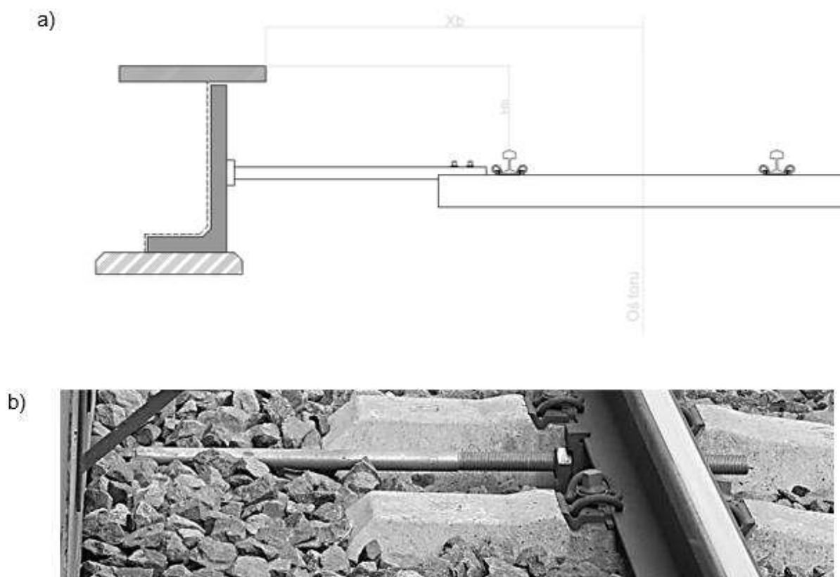
Rys 7 Przykład zabudowy urządzenia zapewniające niezmiennność położenia osi toru względem obiektów stałych (przykładowe rozwiązanie)
