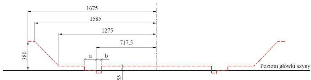
Tablica 8. Poszerzenia części dolnej skrajni budowli (dla wysokości \leq 380 mm) 1)
