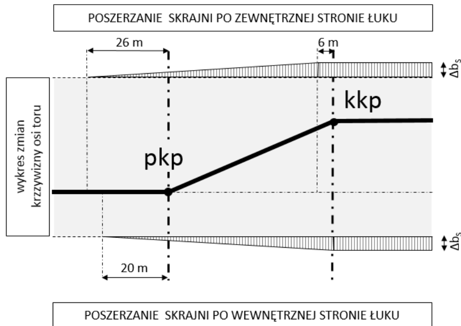
Rys. 3 Zmiany poszerzeń Granicznej Skrajni Zabudowy w konfiguracji prosta-krzywa przejściowa – łuk poziomy
