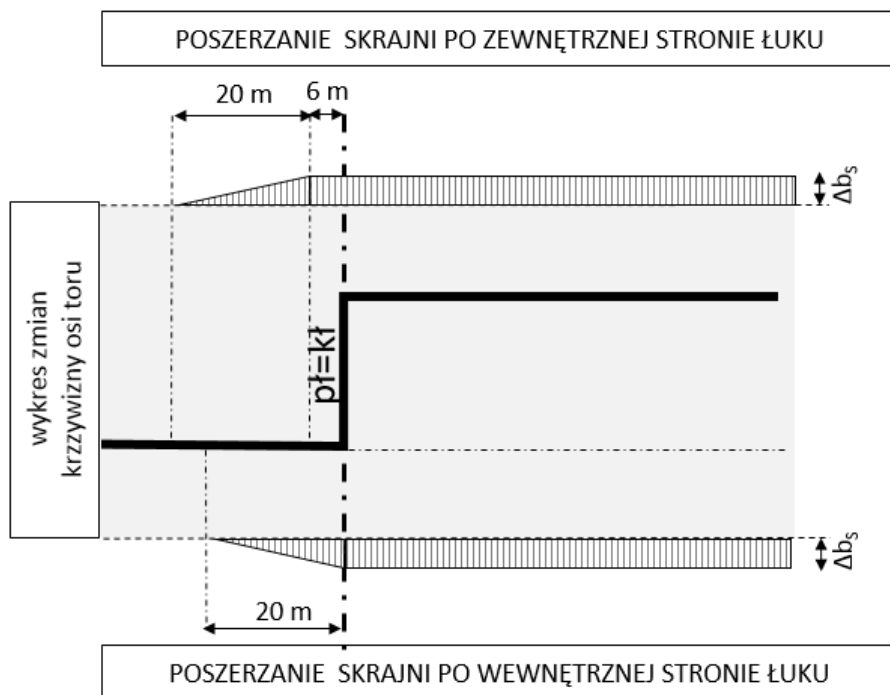
Rys. 4 Zasady zmiany poszerzeń Granicznej Skrajni Zabudowy w konfiguracji prosta – łuk poziomy
