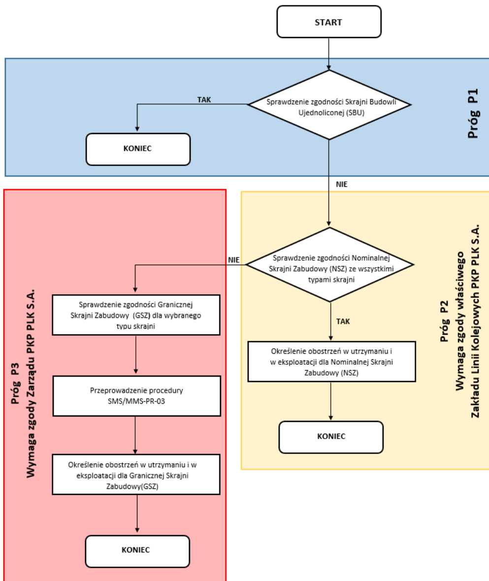
Rys. 1 Schemat postępowania w przypadku niezachowania Skrajni Budowli Ujednoliconej (SBU)
