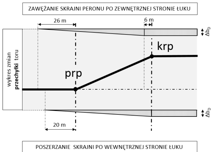
Rys. 5 Zasady zmian poszerzeń i zwężeń skrajni Granicznej Skrajni Zabudowy z uwagi na zmiany przechyłki toru
