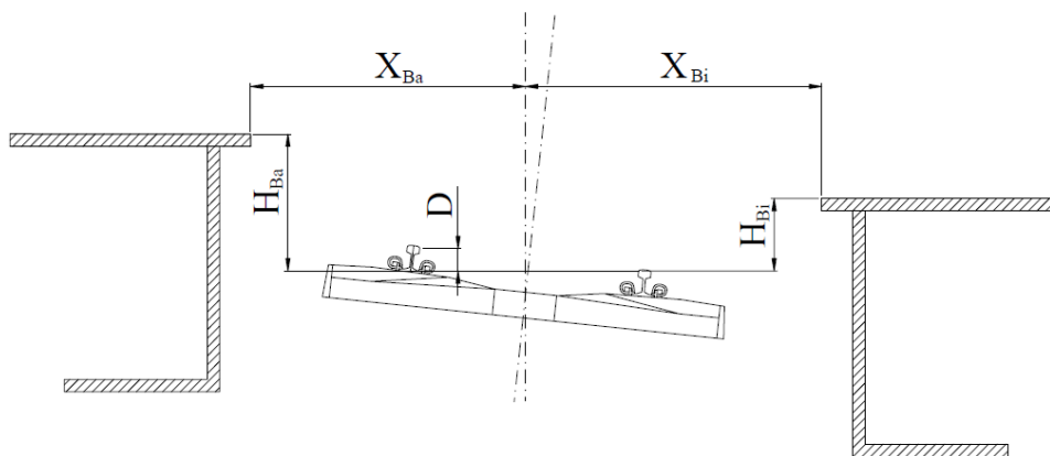
Rys. 2 Wpływ krzywizny łuku i przechyłki toru na wysokość peronu oraz odległość krawędzi peronu od osi toru
