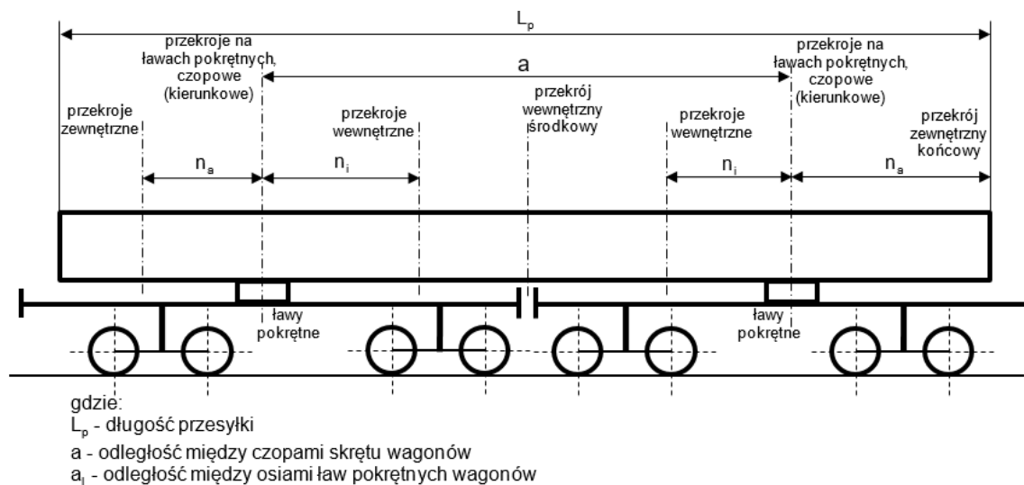
Rys. 7.2 Schemat przekrojów przesyłki załadowanej na dwa wagony z ławami pokrętnymi
