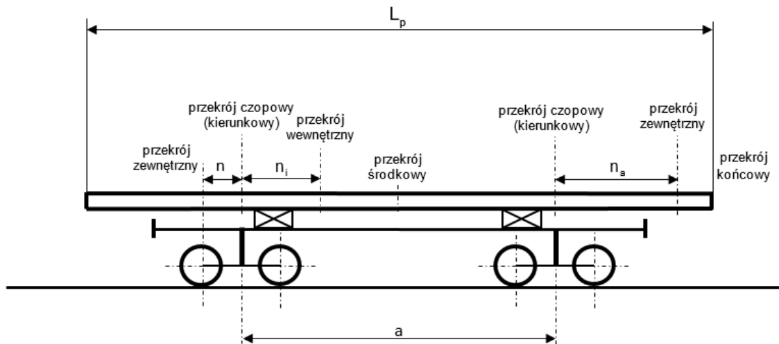
Rys. 7.2 Schemat przekrojów przesyłki załadowanej na dwa wagony z ławami pokrętnymi
