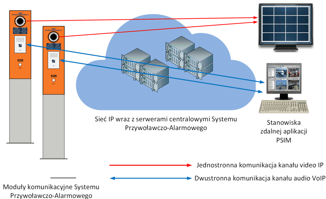
Rys. 3. Schemat ogólnej architektury systemu Przywoławczo-Alarmowego
