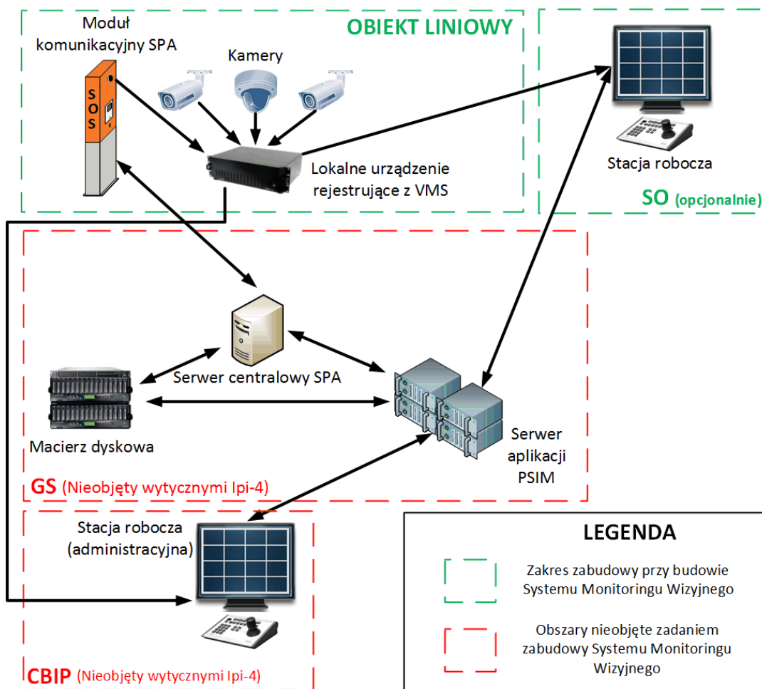
Rys. 1. Schemat logiczny SMW wraz z podsystemem SPA
