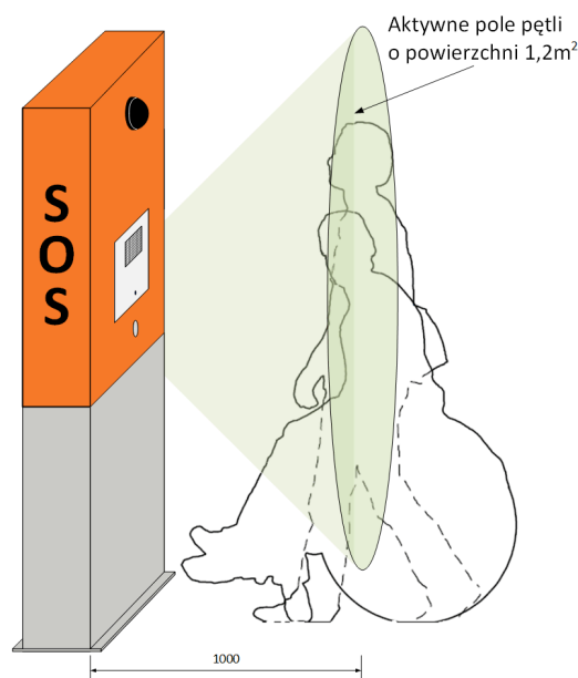
Rys. 7. Obszar prawidłowego odsłuchu dla modułu komunikacyjnego SPA
