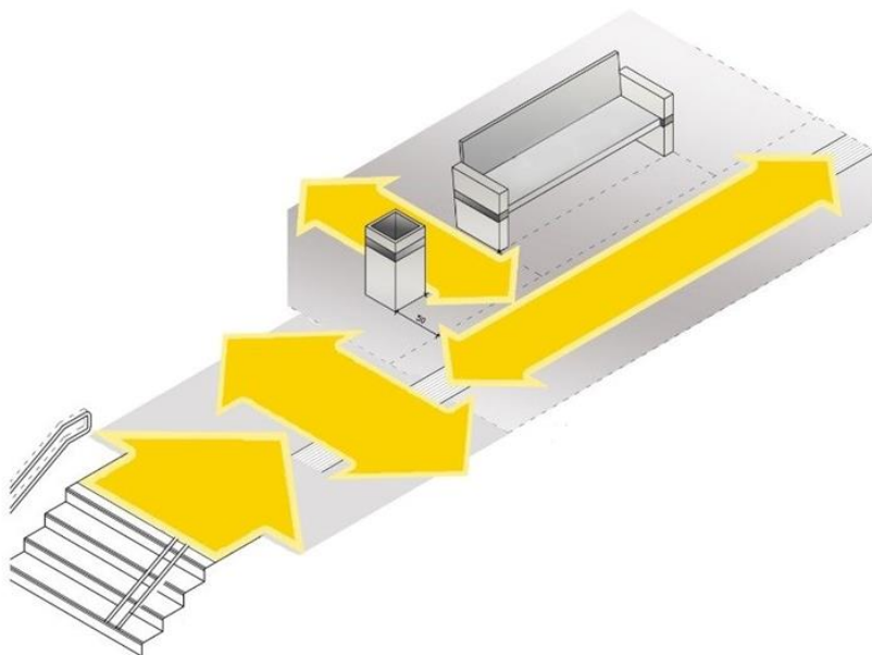
Rysunek 13 Zalecane minimalne odległości między elementami wyposażenia peronu (rys. opracowano na podstawie materiałów własnych)
