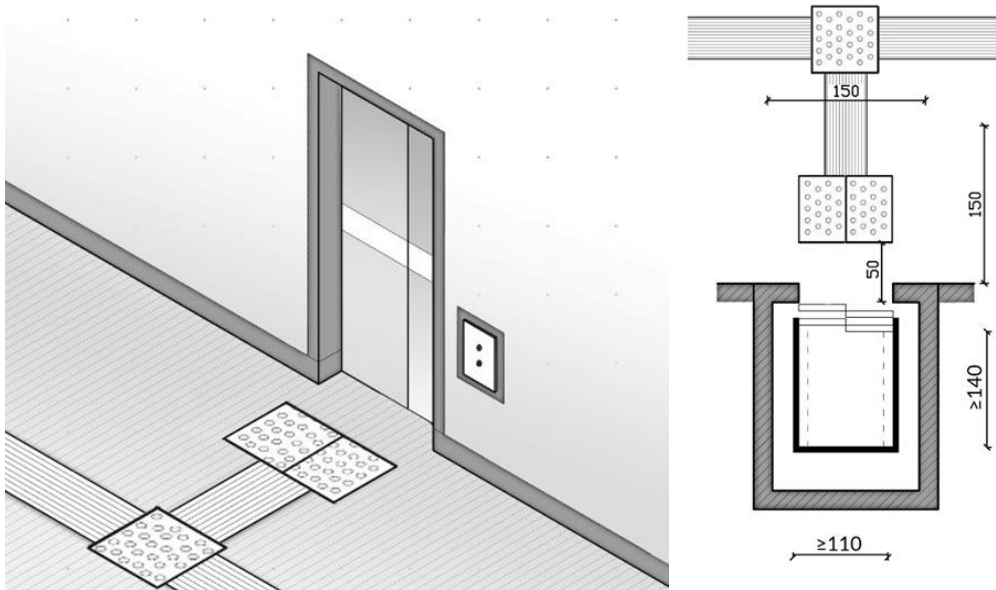
Rysunek 29 Ścieżka prowadząca oraz pas ostrzegawczy przed windą (rys. opracowano na podstawie materiałów własnych)
