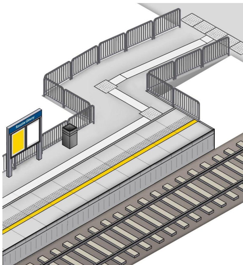
Rysunek 23 Przykładowe wejście na peron jednokrawędziowy (rys. opracowano na podstawie materiałów własnych)
