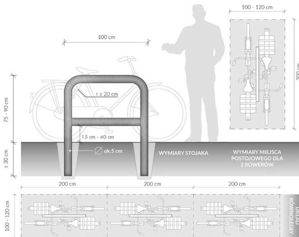
Rysunek 33 Wymiary stojaka rowerowego oraz miejsc postojowych dla rowerów (rys. opracowano na podstawie materiałów własnych)
