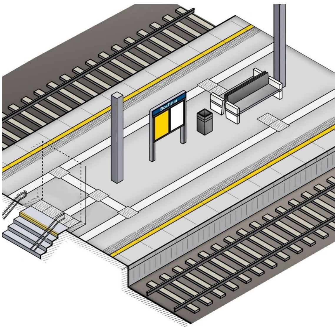
Rysunek 19 Przykład peronu wyposażonego w pełne oznakowanie dotykowe (rys. opracowano na podstawie materiałów własnych)
