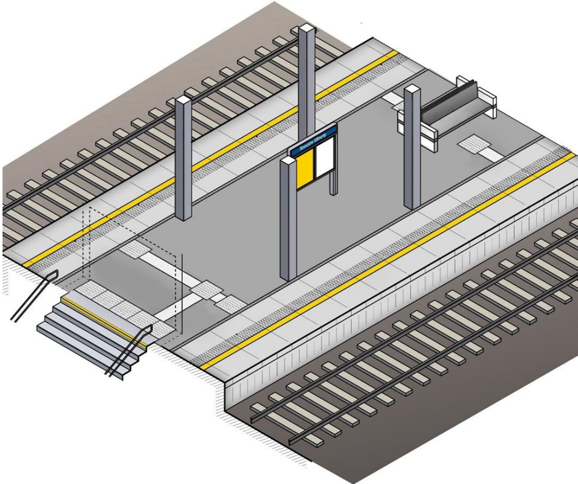
Rysunek 18 Przykład peronu, na którym system oznakowania dotykowego należy do wzoru ostrzegawczego wskazującego na zagrożenie na granicy strefy zagrożenia. (rys. opracowano na podstawie materiałów własnych)
