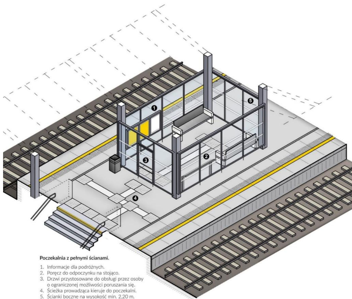
Rysunek 31 Poczekalnia pod wiatą z pełnymi ścianami (rys. opracowano na podstawie materiałów własnych)
