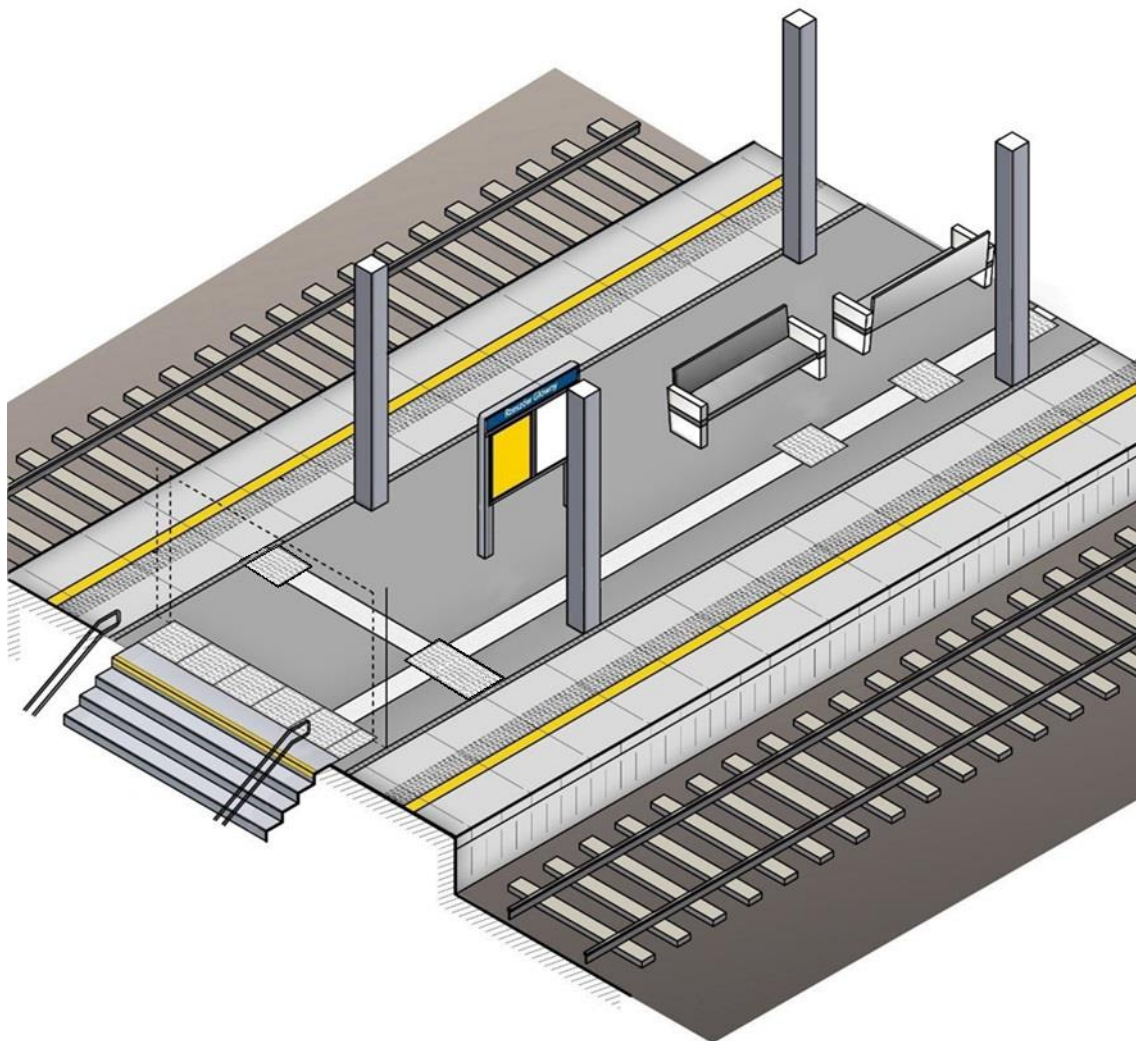
Rysunek 20 Przykład peronu z przerwanymi ścieżkami prowadzącymi – zakończonymi polem uwagi znajdującym się w odległości 0,5 m od przeszkody (rys. opracowano na podstawie materiałów własnych)
