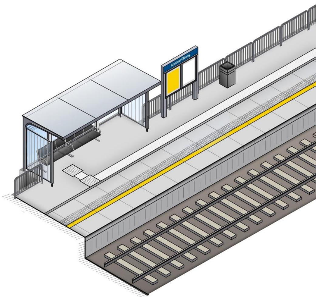
Rysunek 15 Zalecane zagospodarowanie peronu jednokrawędziowego (rys. opracowano na podstawie materiałów własnych)
