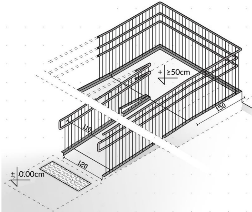
Rysunek 28 Pochylnia z różnicą wysokości \geq 0,5 m wyposażona w poręcze na wysokości 0,75 m i 0,9 m oraz w pochwyty na wysokości 1,1 m (rys. opracowano na podstawie Rozporządzenia Ministra Transportu i Gospodarki Morskiej z dnia 30 maja 2000 r. w sprawie warunków technicznych, jakim powinny odpowiadać drogowe obiekty inżynierskie i ich usytuowanie (Dz. U. z 2000 r. poz. 735, z późn. zm))
