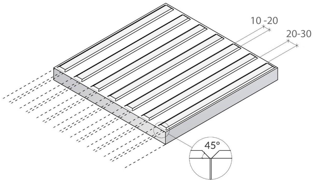
Rysunek 17 Płytki ścieżki prowadzącej (rys. opracowano na podstawie materiałów własnych)
