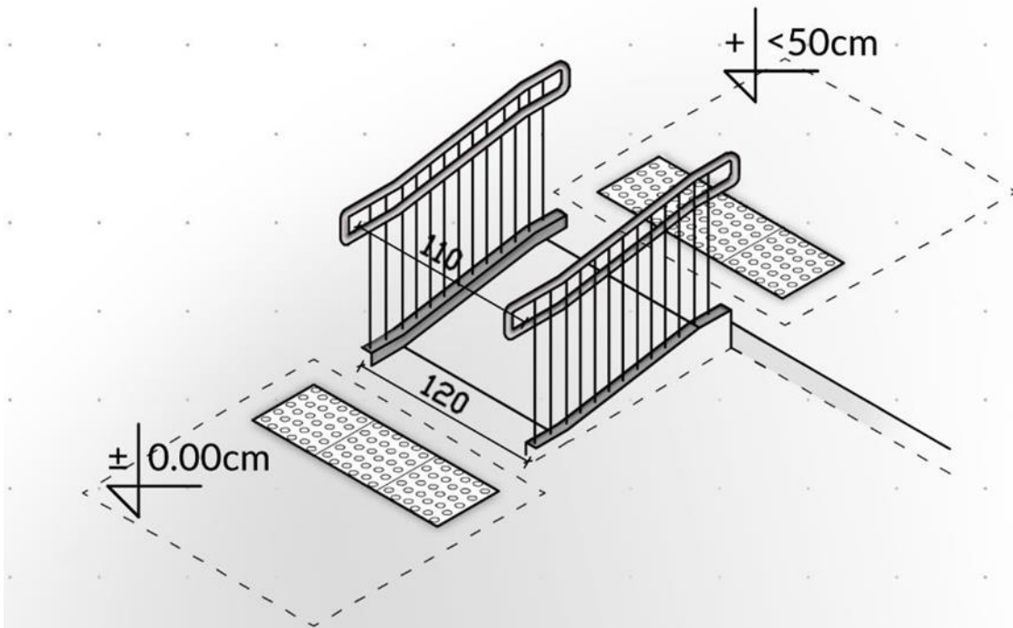
Rysunek 27 Pochylnia z różnicą wysokości < 0,5 m wyposażona w poręcze na wysokości 0,75 m i 0,9 m
