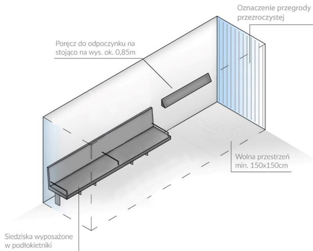
Rysunek 30 Przykładowe wyposażenie wiaty jednostronnej (rys. opracowano na podstawie materiałów własnych)
