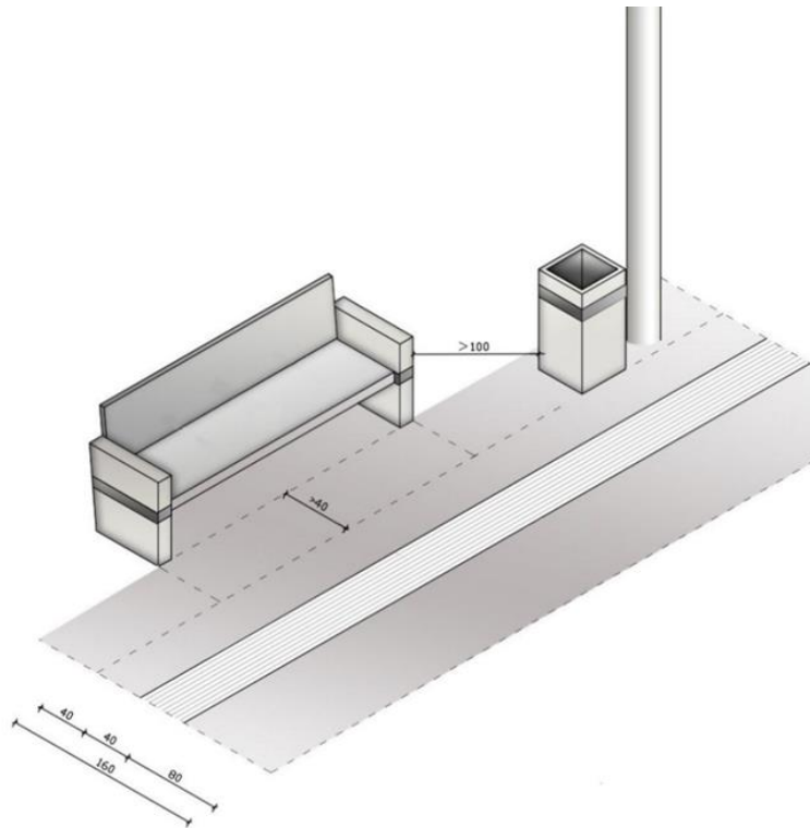
Rysunek 13 Zalecane minimalne odległości między elementami wyposażenia peronu (rys. opracowano na podstawie materiałów własnych)
