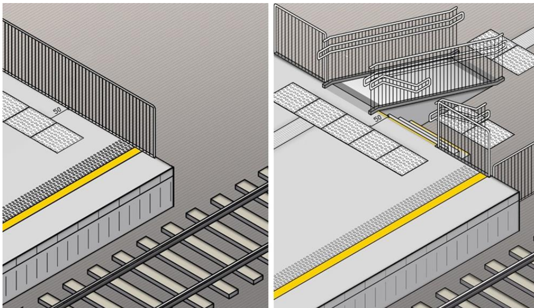
Rysunek 22 Przykładowe zakończenia peronów (rys. opracowano na podstawie materiałów własnych)
