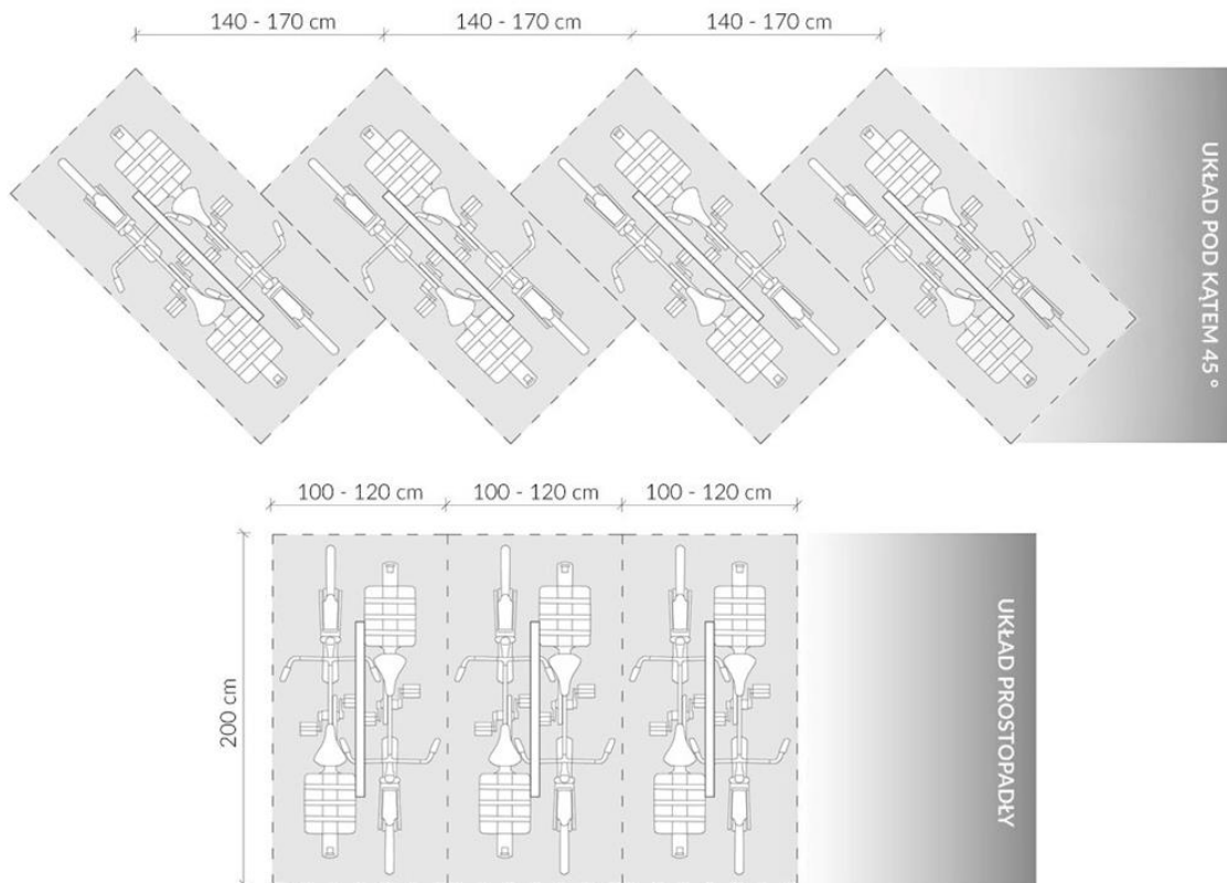
Rysunek 34 Przykładowe układy miejsc postojowych dla rowerów (rys. opracowano na podstawie materiałów własnych)
