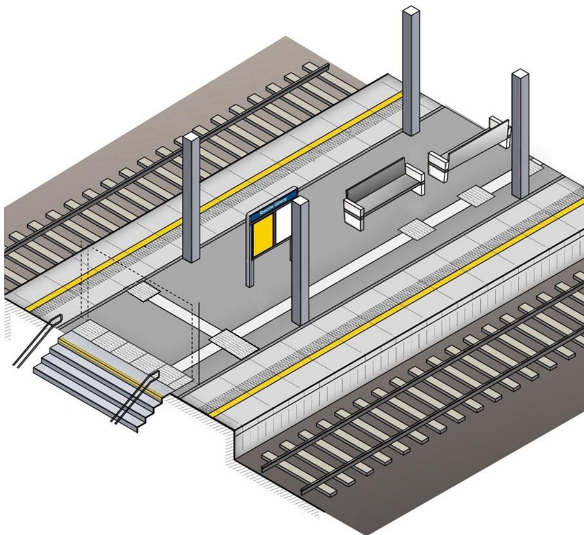
Rysunek 20 Przykład peronu z przerwanyi ścieżkami prowadzącymi – zakończonymi polem uwagi znajdującym się w odległości 0,5 m od przeszkody (rys. opracowano na podstawie materiałów własnych)
