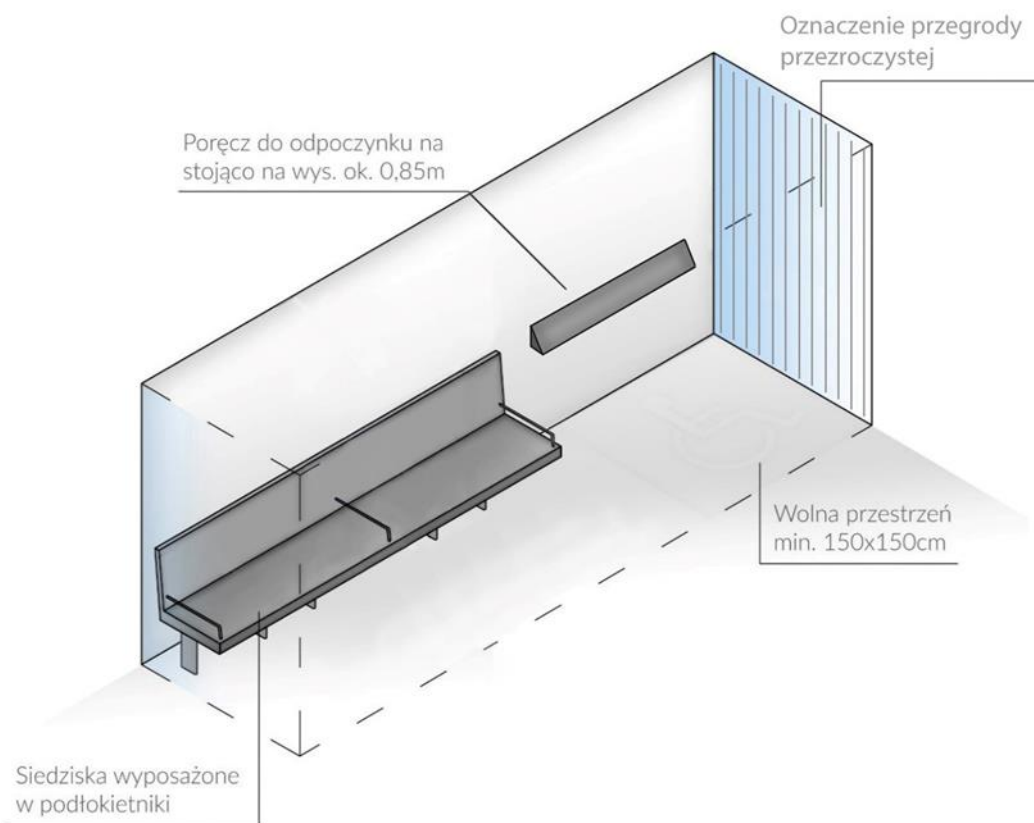
Rysunek 30 Przykładowe wyposażenie wiaty jednostronnej (rys. opracowano na podstawie materiałów własnych)
