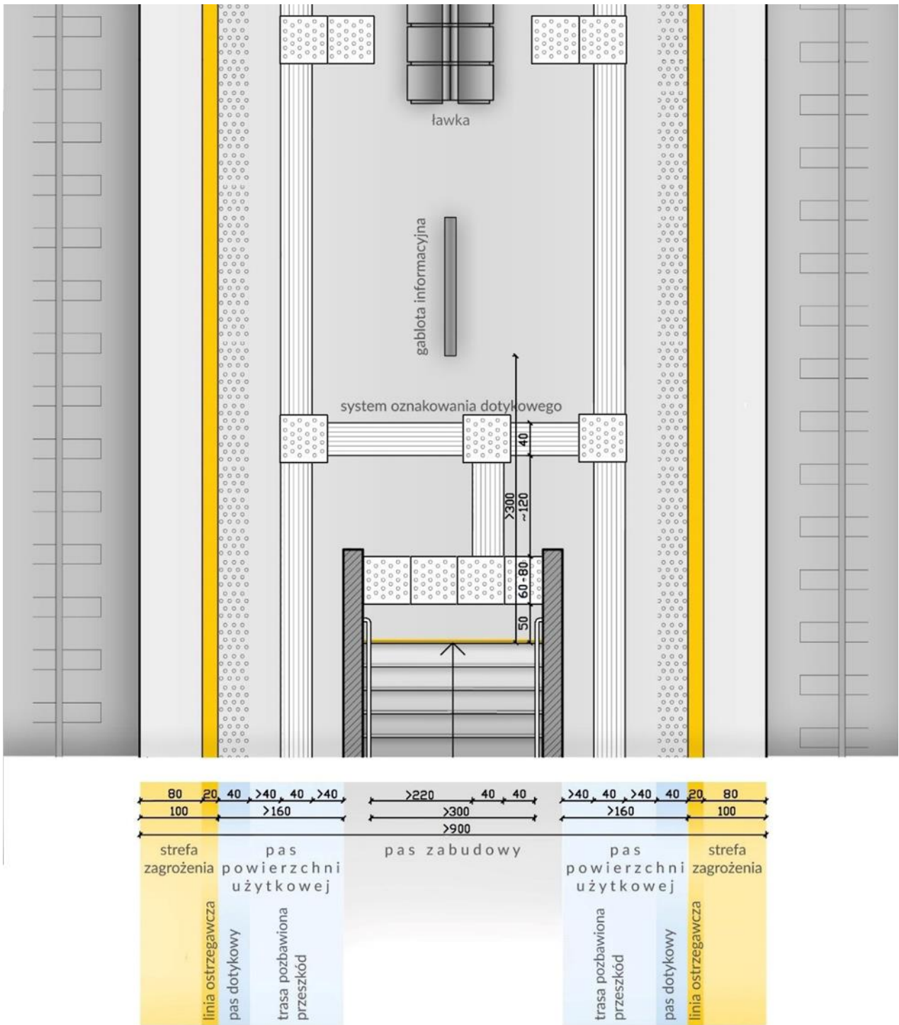
Rysunek 10 Przykład oznakowania dotykowego w nawierzchni peronu przystosowanego do prędkości 60 \text{ km/h} < v < 140 \text{ km/h} (rys. opracowano na podstawie TSI PRM oraz Rozporządzenie Ministra Transportu i Gospodarki Morskiej z dnia 10 września 1998 r. w sprawie warunków technicznych, jakim powinny odpowiadać budowle kolejowe i ich usytuowanie (Dz.U. poz. 987 z późn. zm.))
