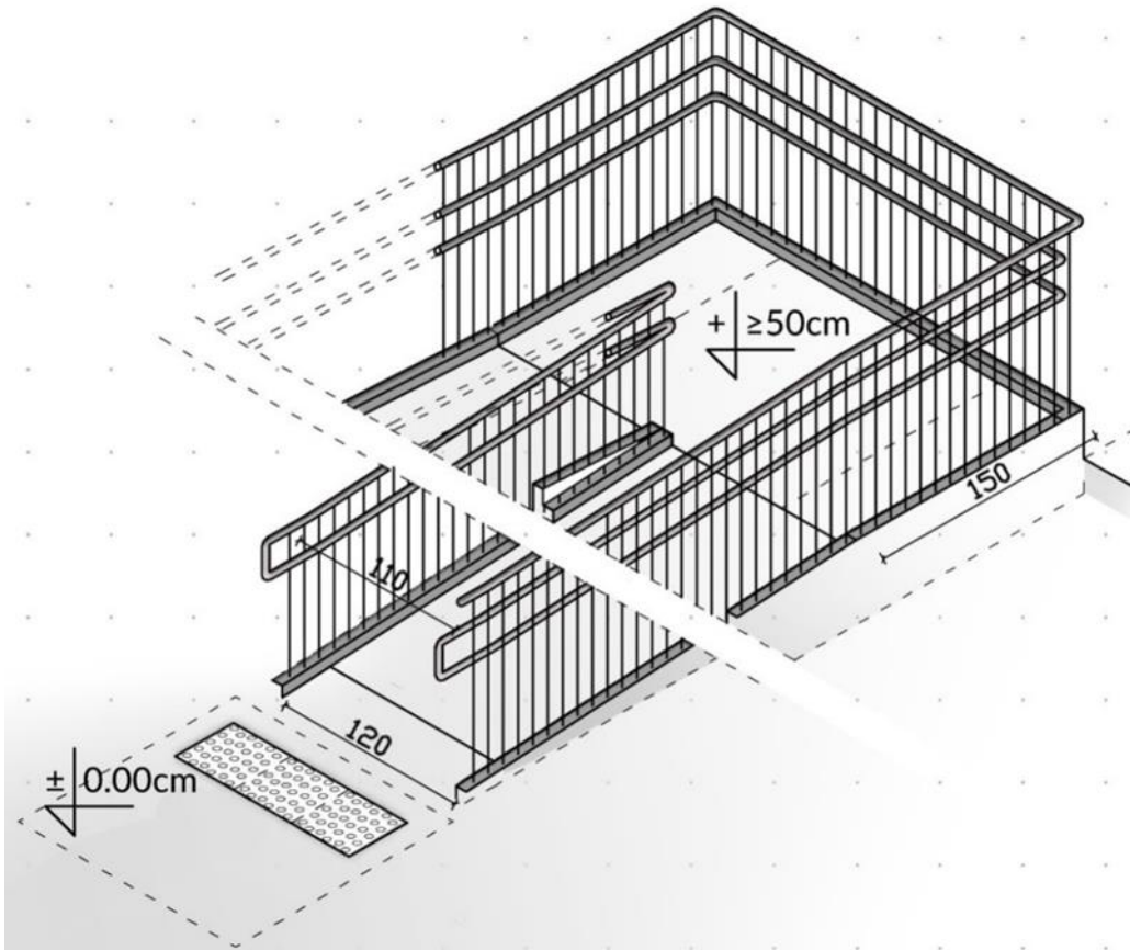
Rysunek 28 Pochylnia z różnicą wysokości \geq 0,5 m wyposażona w poręczę na wysokości 0,75 m i 0,9 m oraz w pochwyt na wysokości 1,1 m (rys. opracowano na podstawie Rozporządzenia Ministra Transportu i Gospodarki Morskiej z dnia 30 maja 2000 r. w sprawie warunków technicznych, jakim powinny odpowiadać drogowe obiekty inżynierskie i ich usytuowanie (Dz. U. z 2000 r. poz. 735, z późn. zm)
