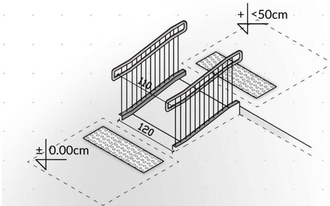
Rysunek 27 Pochylnia z różnicą wysokości < 0,5 m wyposażona w poręcze na wysokości 0,75 m i 0,9 m
