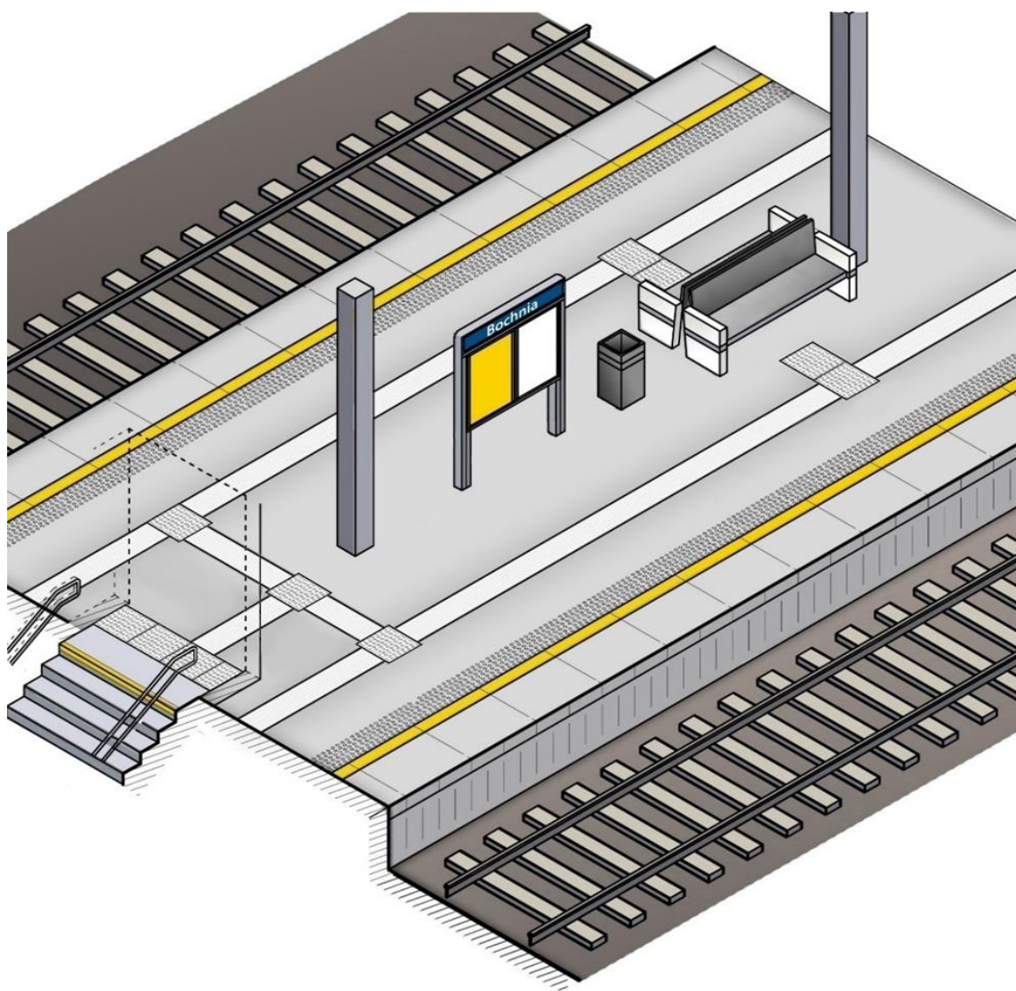
Rysunek 19 Przykład peronu wyposażonego w pełne oznakowanie dotykowe (rys. opracowano na podstawie materiałów własnych)
