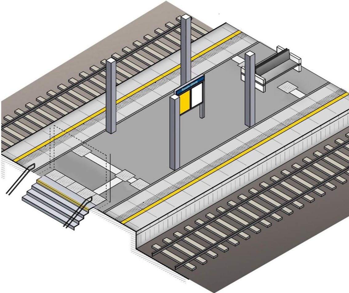
Rysunek 18 Przykład peronu, na którym system oznakowania dotykowego należy do wzoru ostrzegawczego wskazującego na zagrożenie na granicy strefy zagrożenia. (rys. opracowano na podstawie materiałów własnych)
