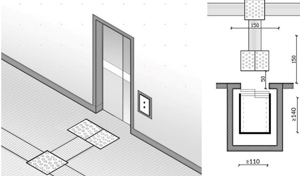
Rysunek 29 Ścieżka prowadząca oraz pas ostrzegawczy przed windą (rys. opracowano na podstawie materiałów własnych)
