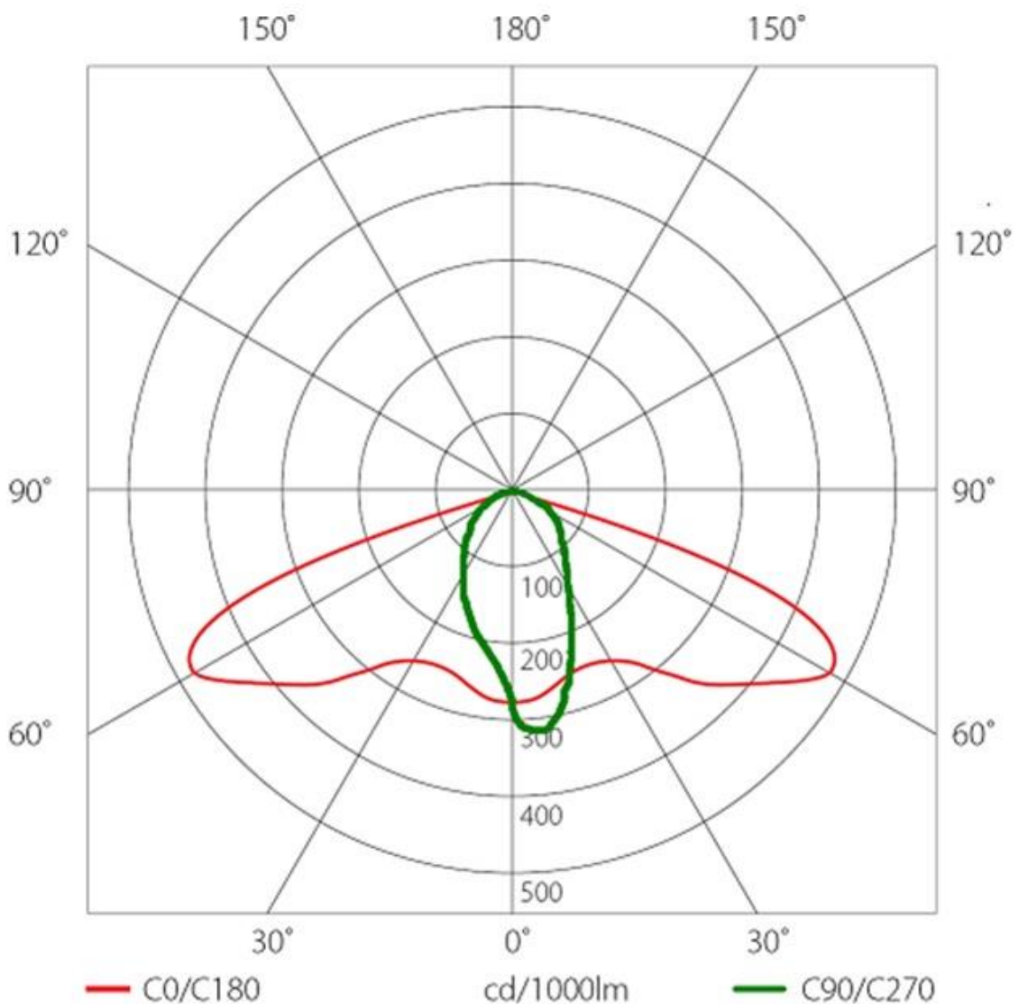
Teoretyczny wykres światłości dla oprawy oświetleniowej
