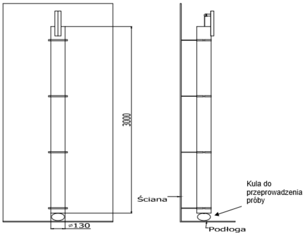
Rysunek 4 Przykładowe stanowisko pomiarowe
