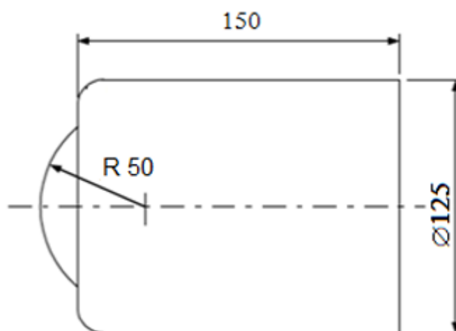
Rysunek 2. Przykładowy model młotka wykorzystywanego w próbie badania odporności na uderzenia mechaniczne min. 140 J, masa 10 kg.
