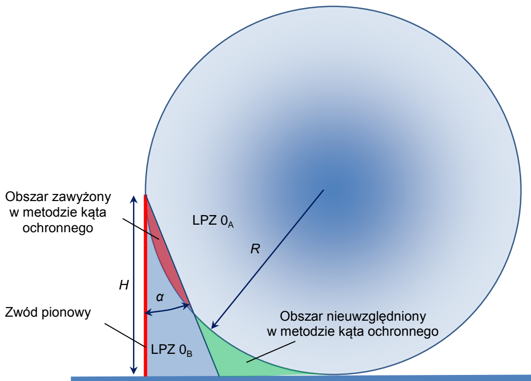
Rys. 5.2.1. Porównanie metod kąta ochronnego i toczonej się kuli, gdzie: \alpha - kąt ochronny, R – promień toczonej kuli
