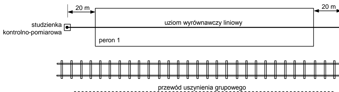
Rys. 2.7.4. Usytuowanie uziumu wyrównawczego na peronie stacji osobowej
