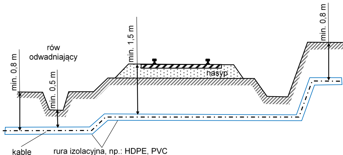
Rys. 6.4.1. Wykonanie przepustów kablowych pod torami
