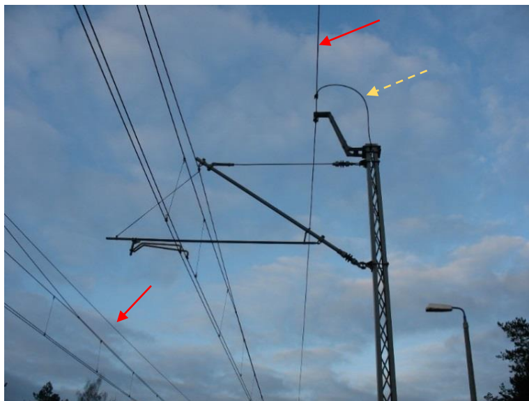
Rys. 4.6.1. Przewody uszynienia grupowego nad siecią trakcyjną DC 3 kV (na górnym zdjęciu z lewej strony strzałką niebieską z linią przerywaną wskazano linię niezmodernizowaną, wykonaną w systemie uszynienia bezpośredniego - bez przewodu uszynienia grupowego)
