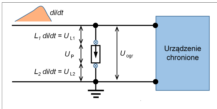
Rys. 4.9.1. Napięcie ograniczania rzeczywistego układu z ogranicznikiem przepięć
