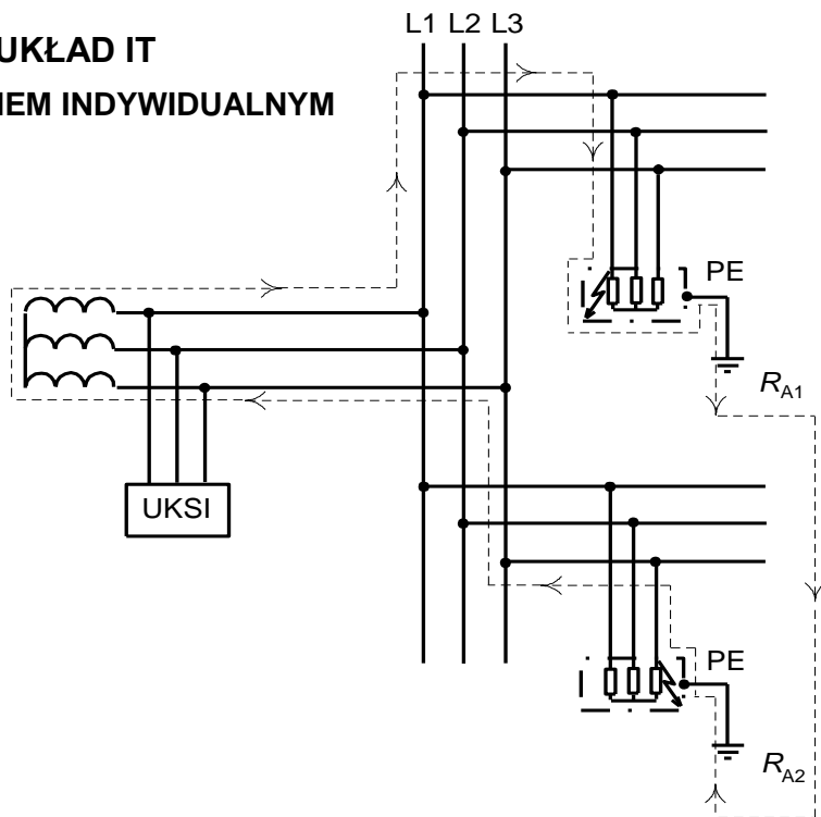
Rys. 2.8.4. Przepływ prądu w układzie IT (bez przewodu neutralnego) przy dwumiejscowym zwarciu z ziemią, gdzie UKSI – urządzenie do kontroli stanu izolacji
