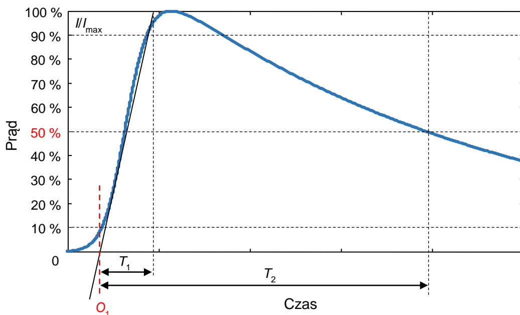
Rys 4.6.3. Definicja parametrów krótkotrwałego impulsu piorunowego (punkt O_1 nazywany jest wirtualnym początkiem udaru krótkotrwałego, wyznaczanym w punkcie przecięcia z osią czasu linii prostej poprowadzonej przez punkty 10 % i 90 % wartości maksymalnej na czole impulsu)
