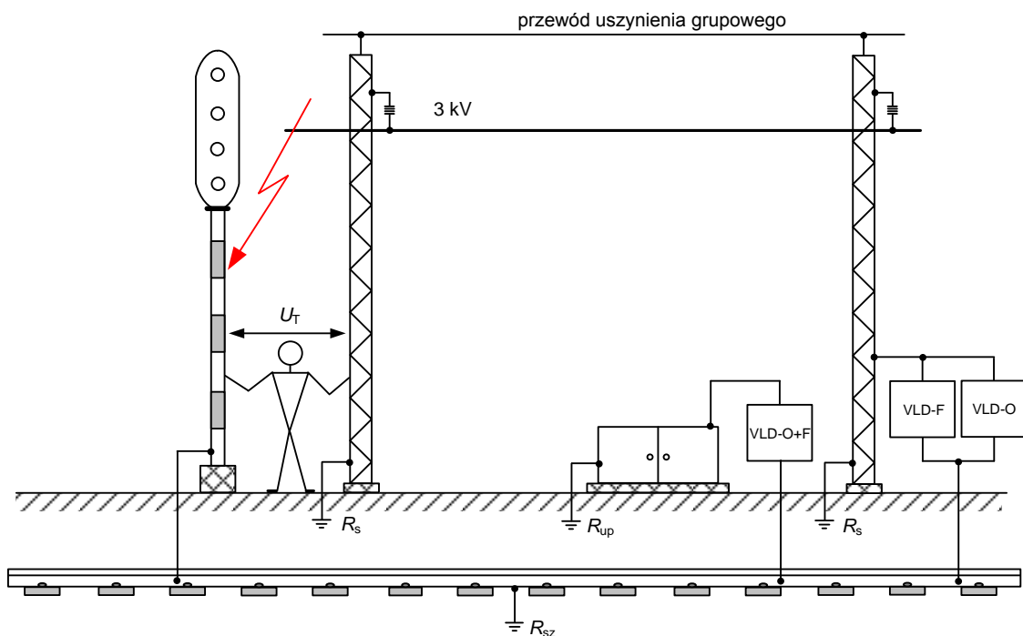
Rys. 2.7.5. Sygnalizator w bezpośrednim pobliżu słupa (w odległości nieprzekraczającej 2,50 m). Stan wyjściowy, bez uzupełniających środków ochrony – napięcie dotykowe U_T o niebezpiecznie dużej wartości utrzymuje się do chwili wyłączenia zasilania w podstacji trakcyjnej
