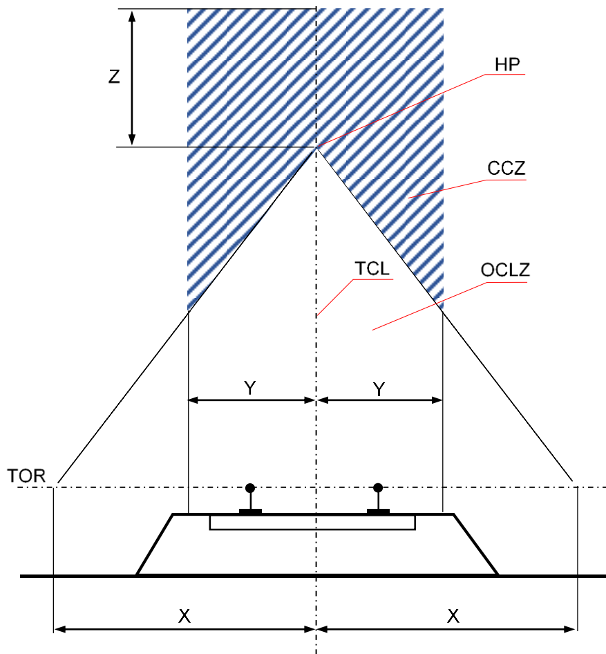
Rys. 2.2.1. Strefa oddziaływania trakcji elektrycznej; strefa górnej sieci jezdnej OCLZ i strefa pantografu CCZ (wg PN-EN 50122-1:2011), gdzie: HP – najwyższy punkt górnej sieci jezdnej, OCLZ – strefa górnej sieci jezdnej, TOR – poziom główki szyny, CCZ – strefa pantografu, TCL – oś toru X = 5,00 \text{ m} Y = 1,7 \text{ m} Z = 0,7 \text{ m}
