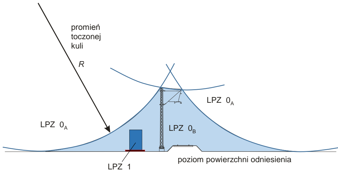
Rys. 5.2.2. Idea wyznaczania stref ochrony odgromowej sieci trakcyjnej
