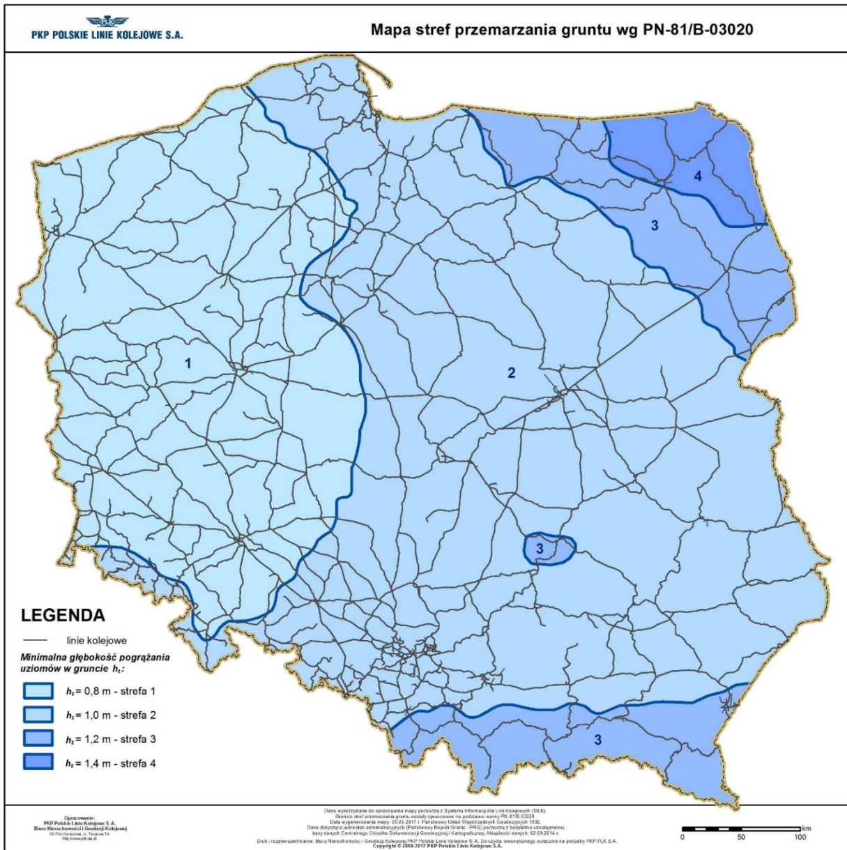
Rys. 5.5.1. Minimalna głębokość pograżania uziomów w gruncie h_z określona na podstawie mapy stref przemarzania gruntu w Polsce wg PN-81/B-03020
