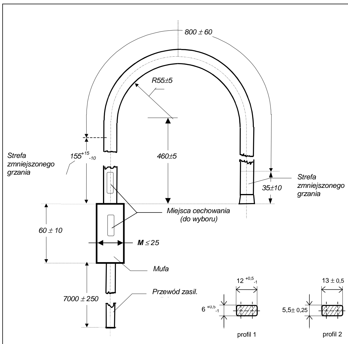
Rys.6. Grzejnik zamknięciowy typu „U” wraz z wymiarami***
