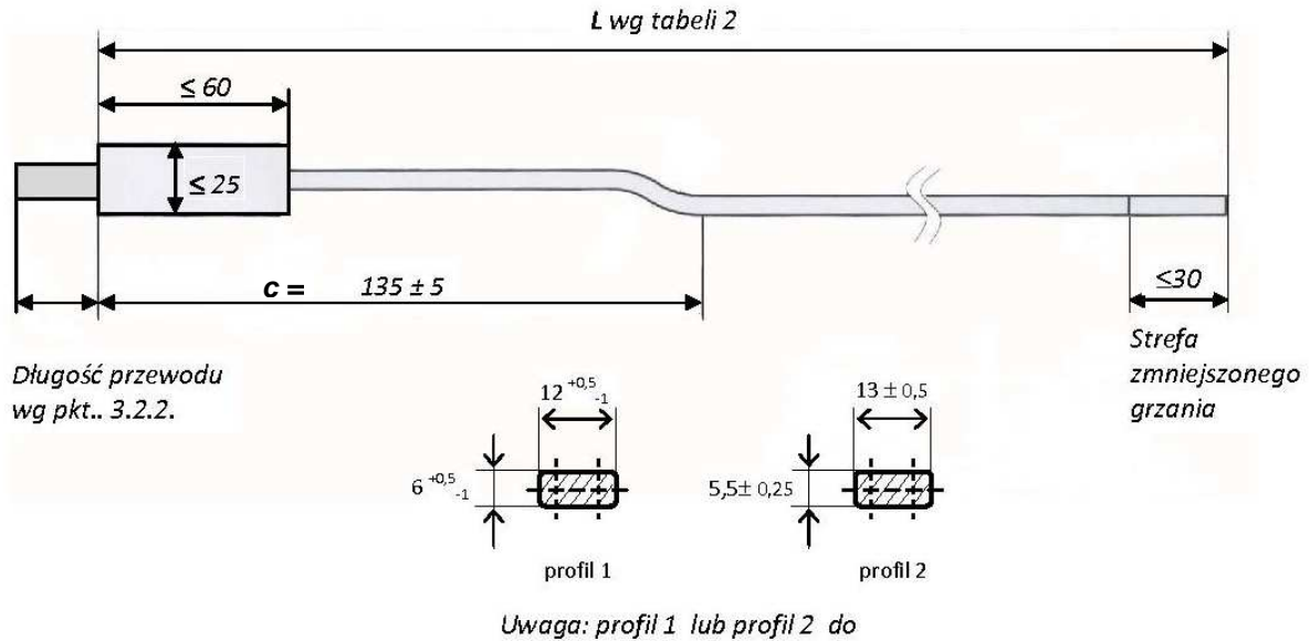
Rys.2. Grzejnik krzyżownicowy wraz z wymiarami
