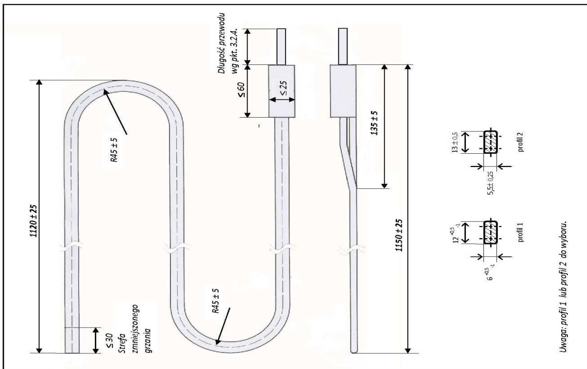
Rys.4. Grzejnik do płyty grzewczej wraz z wymiarami
