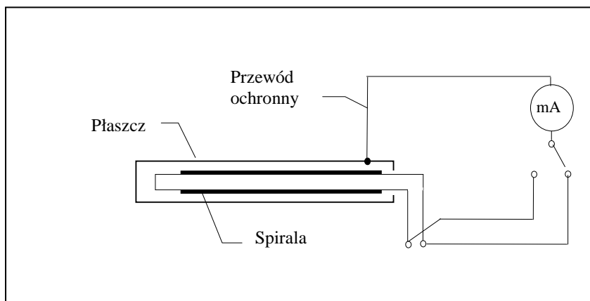
Rys.7. Schemat układu pomiarowego do sprawdzania prądu upływowego (wg PN-EN60335-1:2002)
