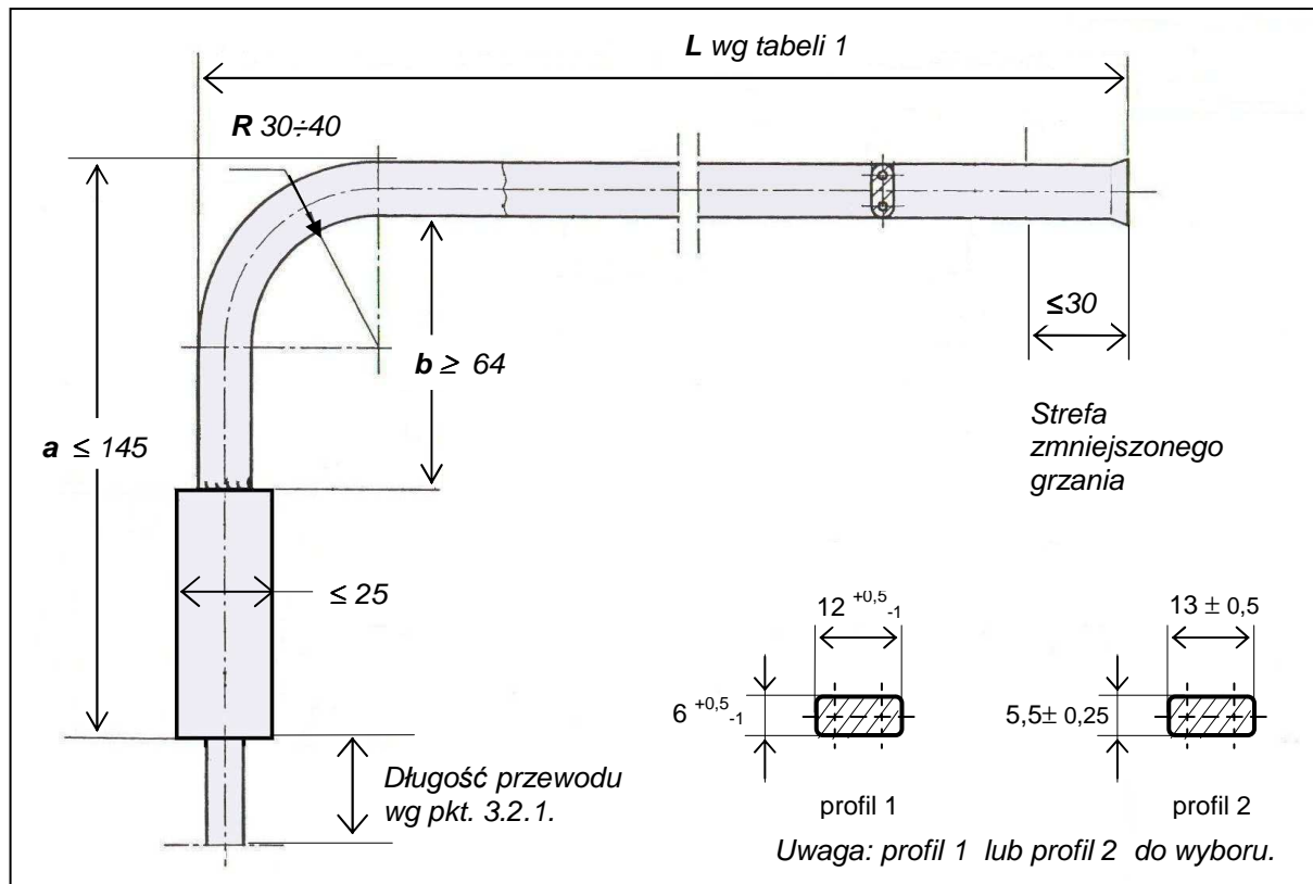
Rys.1. Grzejnik opornicowy wraz z wymiarami
