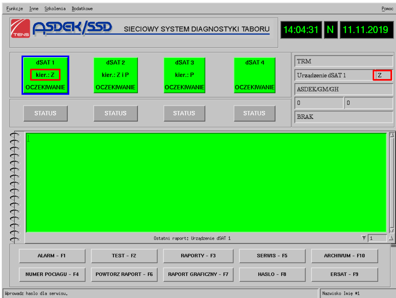
Rysunek 32. Wizualizacja terminala pokazująca rezultat zmian w konfiguracji „Urządzenie dSAT 1”
