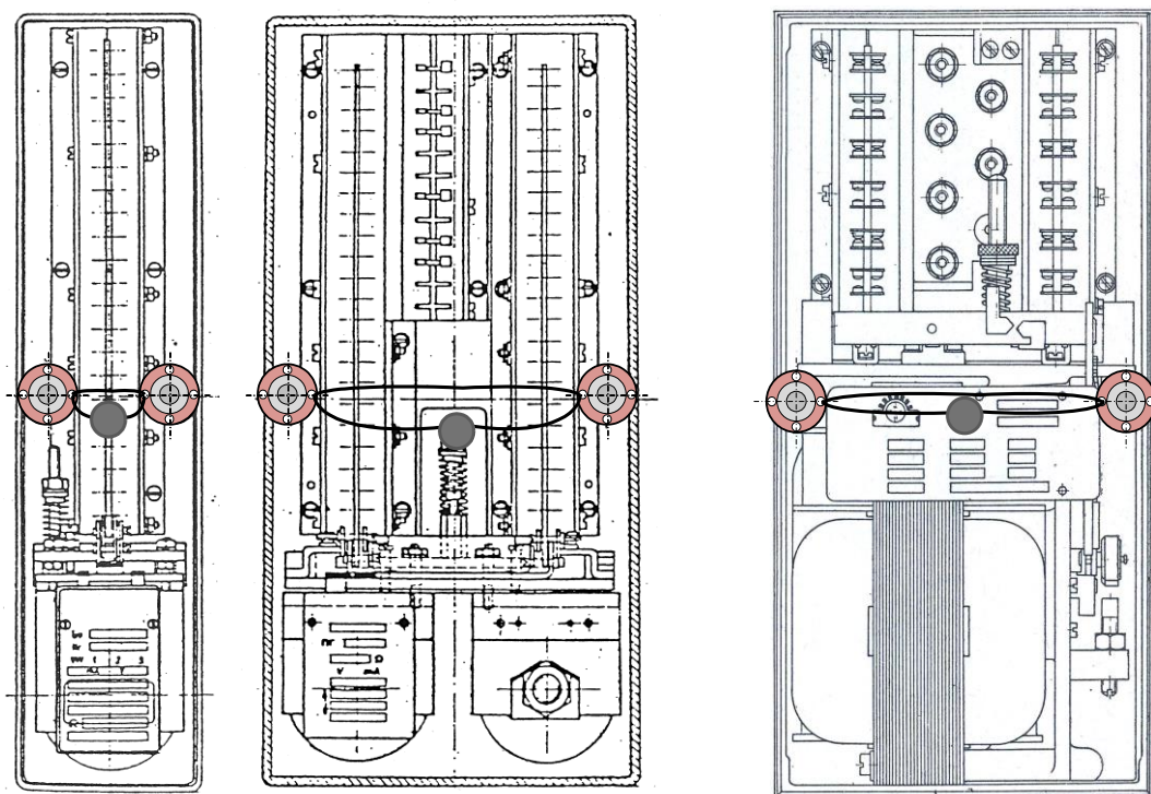
Przełączniki typu JRK, RK, JRJ – widok od czoła
