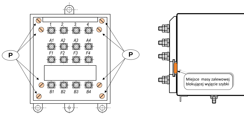
Przekaźniki typu JRG, RG – widok od czola i z boku
