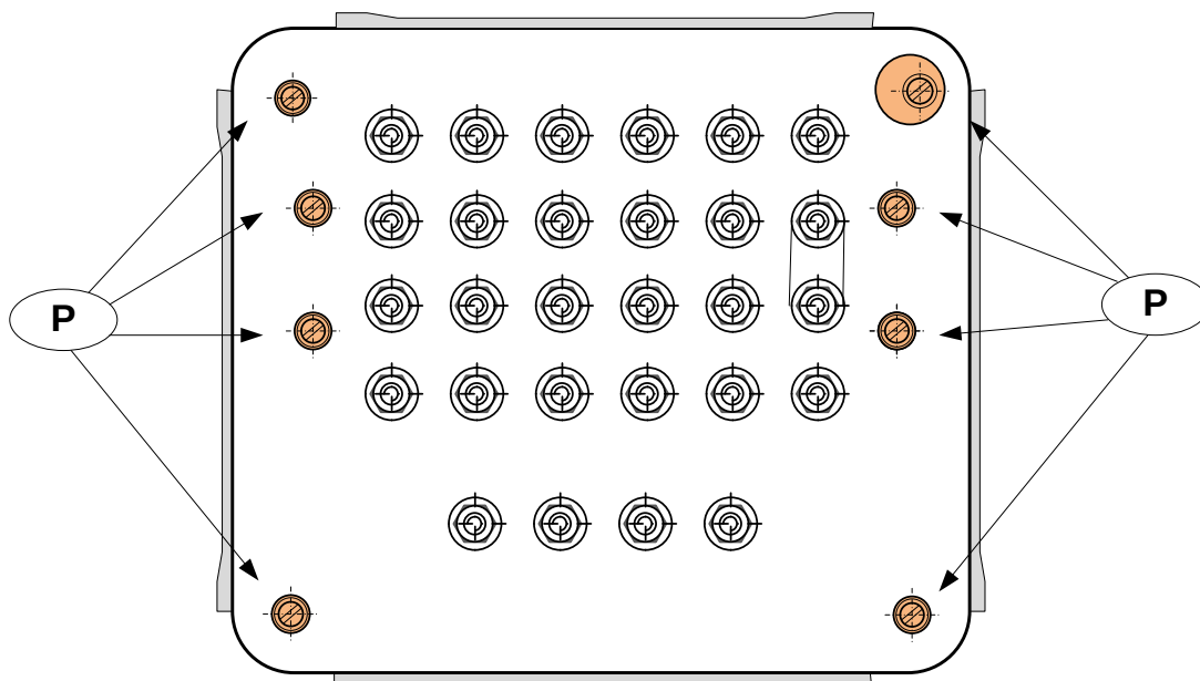
Przekaźniki typu JRV, JRY – widok z góry
