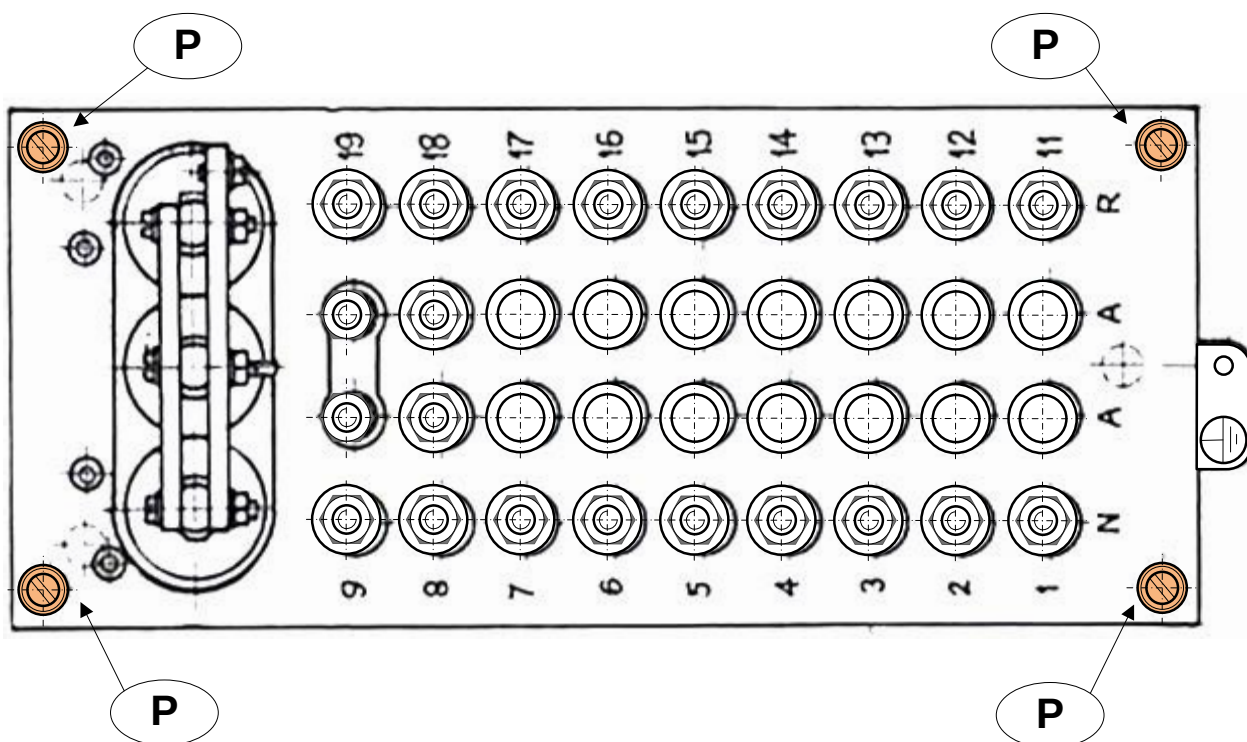
Przekaźniki typu JRR – widok z góry
