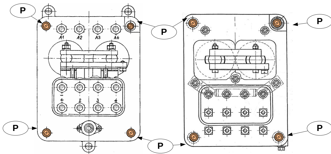
Przekaźniki typu JRC, JRM, RM
