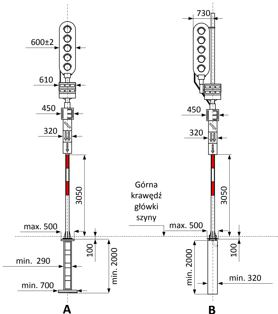
Rysunek 3. Wymiary gabarytowe standardowego sygnalizatora kolejowego świetlnego wysokiego w przykładowej wersji funkcjonalnej umieszczonego na przykładowych, typowych fundamentach: A stalowym (Patrz §15 ust. 3); B palowym sygnalizatora, latarnia sygnałowa umieszczona na wysięgniku
