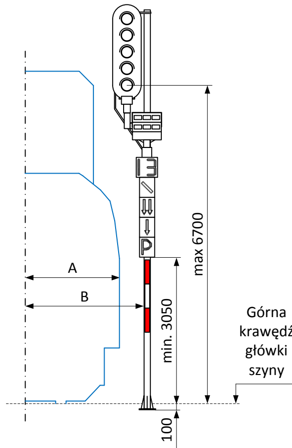
Rysunek 12. Odległość standardowego sygnalizatora kolejowego świetlnego wysokiego od osi toru usytuowanego na ławie torowiska
