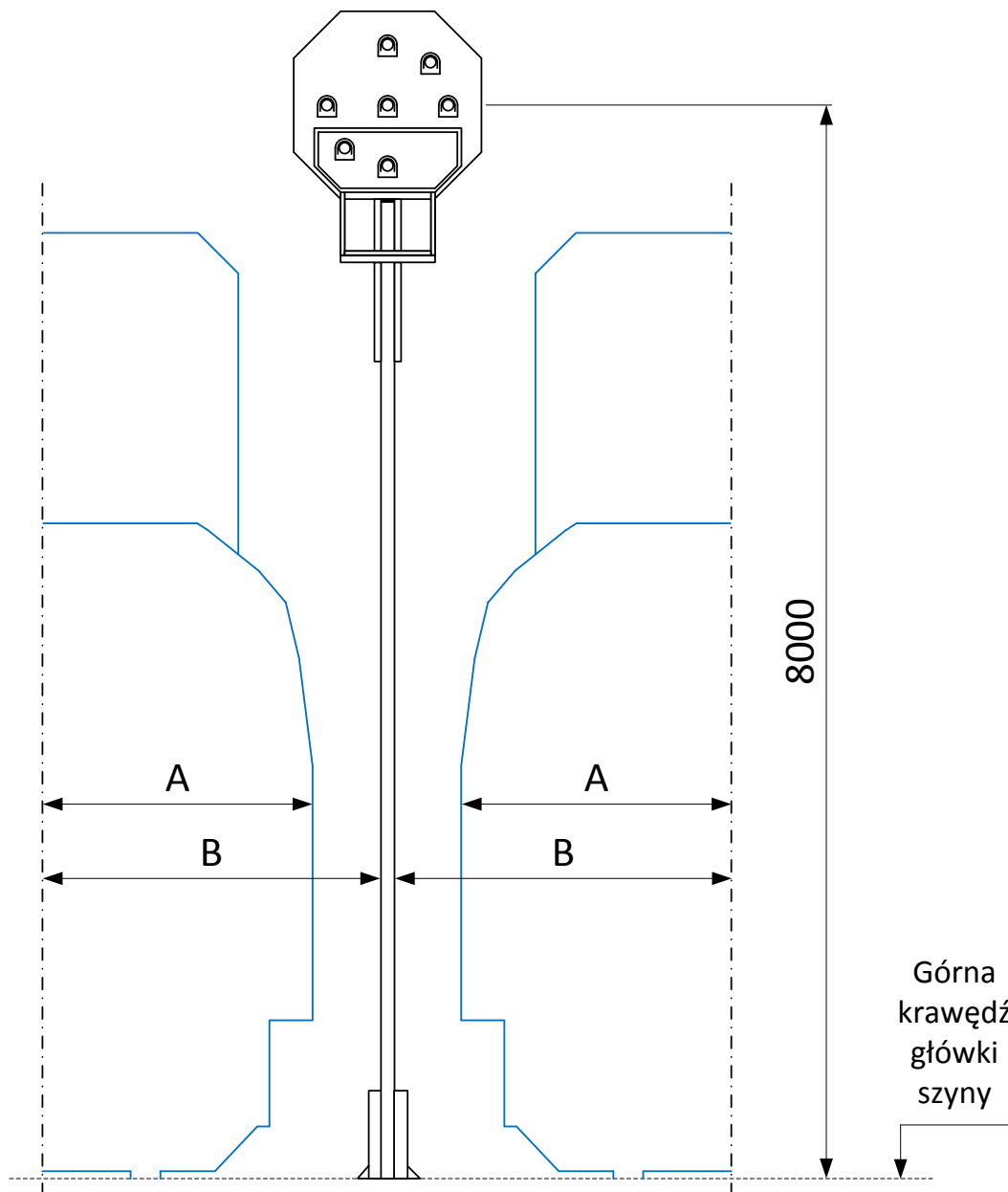
Rysunek 14. Usytuowanie tarczy rozrządowej na górcy rozrządowej.
