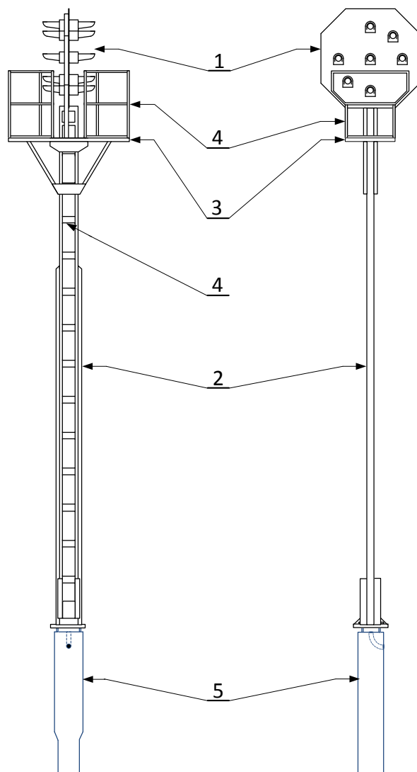
Rysunek 5. Podstawowe elementy składowe tarczy rozrządowej.
