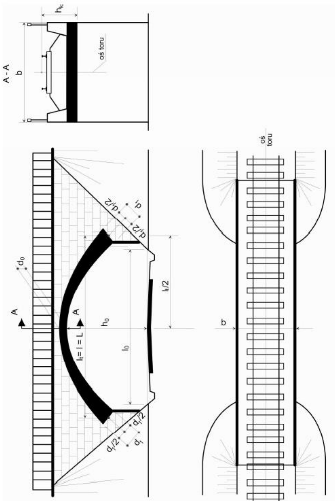
Rys. 2.3. Przekroje i rzut obiektu inżynierskiego o przęśle łukowym sklepionym
