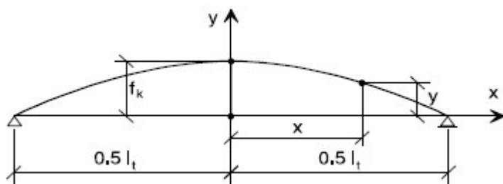
Rys. 3.1. Schemat konstrukcji o schemacie belki swobodnie podpartej
