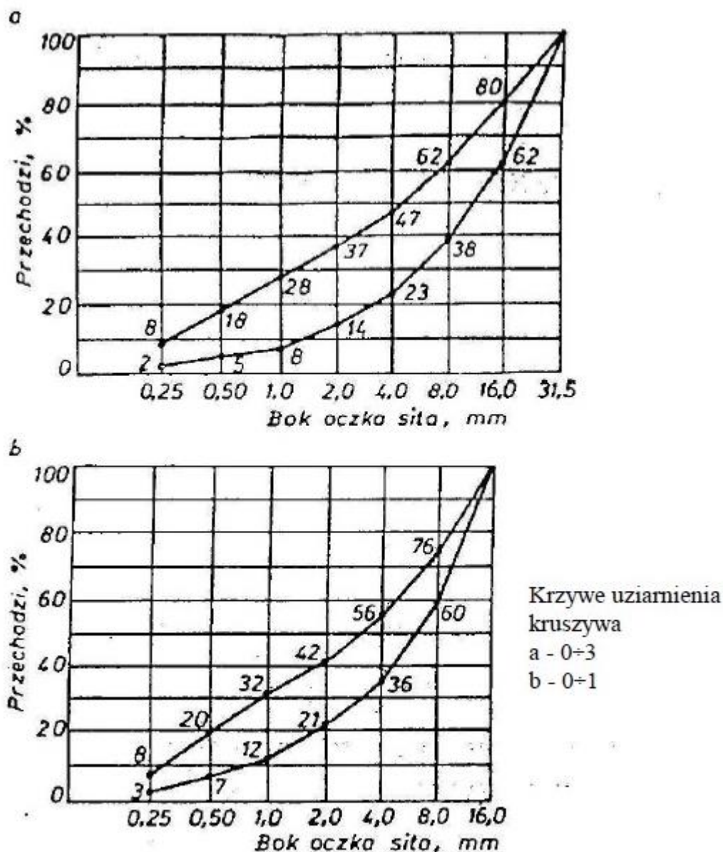
Rys. Z1.1. Graniczne krzywe uziarnienia
