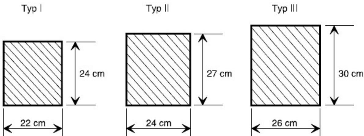
Rys. 3.3. Typy mostownic
