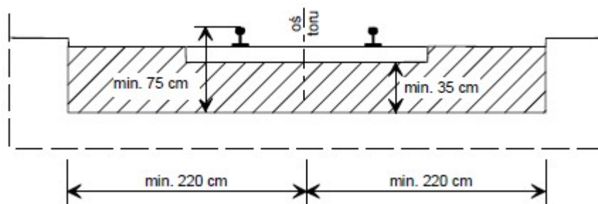
Rys. 3.2. Minimalne wymiary podsypki w obiekcie inżynierskim z torem na podkładach i podsypce
