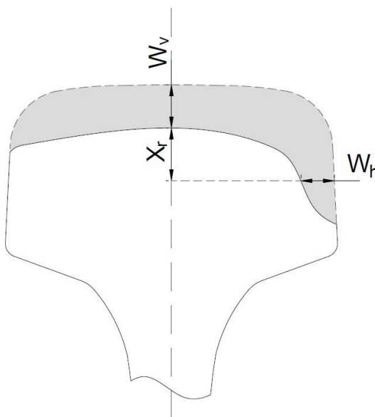
Rys. 1 Pomiar zużycia szyny: W_v – zużycie pionowe, W_h – zużycie boczne, x_r = 15 \text{ mm}
