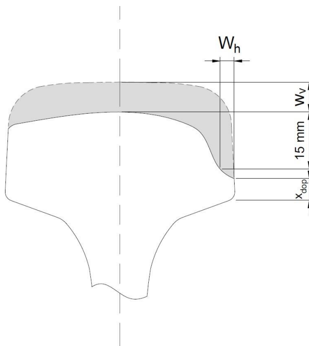
Rys. 2 Pomiar wymiarów poprzecznych szyny staroużytecznej ( W_v , W_h , x_{dop} )
