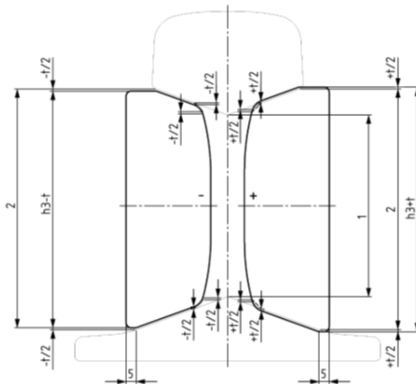
Rysunek 8 Sprawdzenie wysokości komory łukowej
