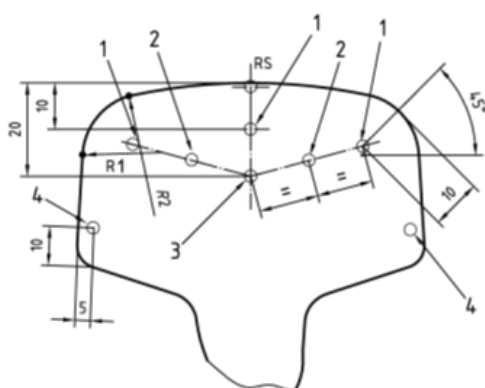
Rys. 7 Miejsca pomiaru twardości.
