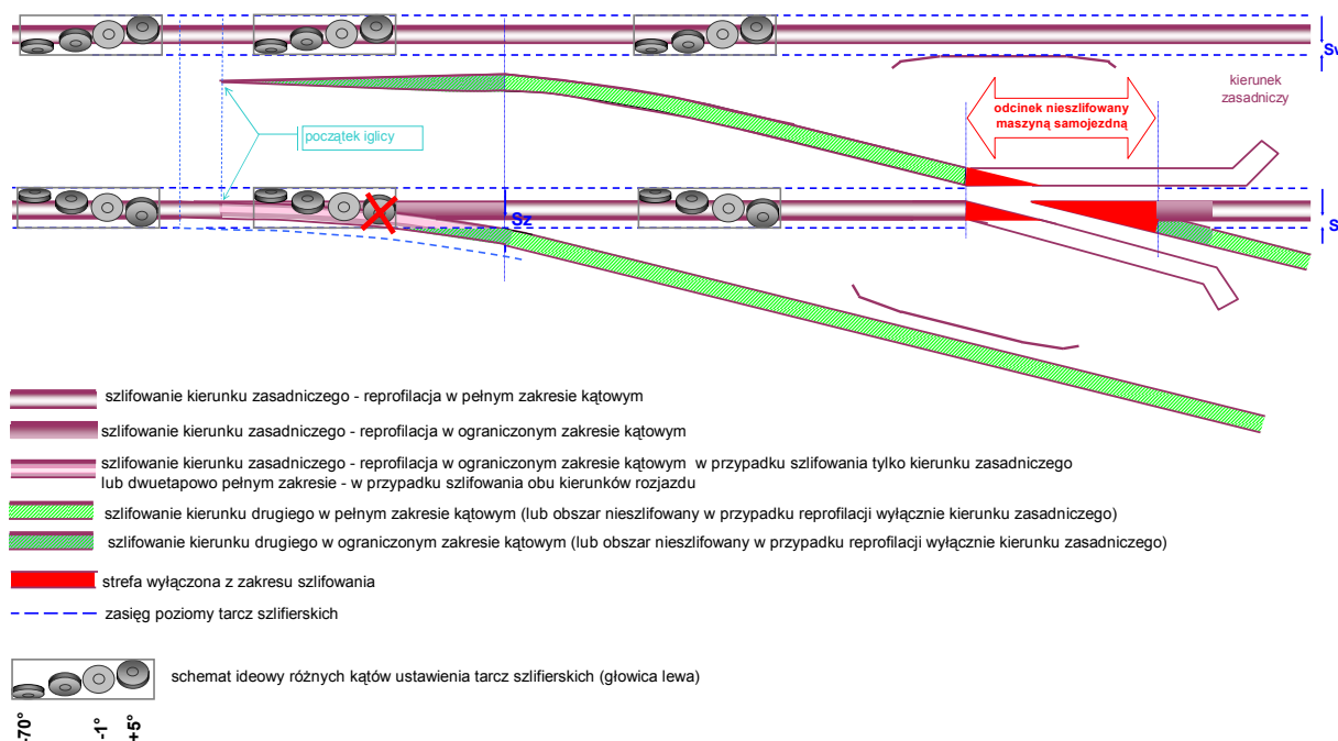
Rys. 4 Schemat stref szlifowania rozjazdu
