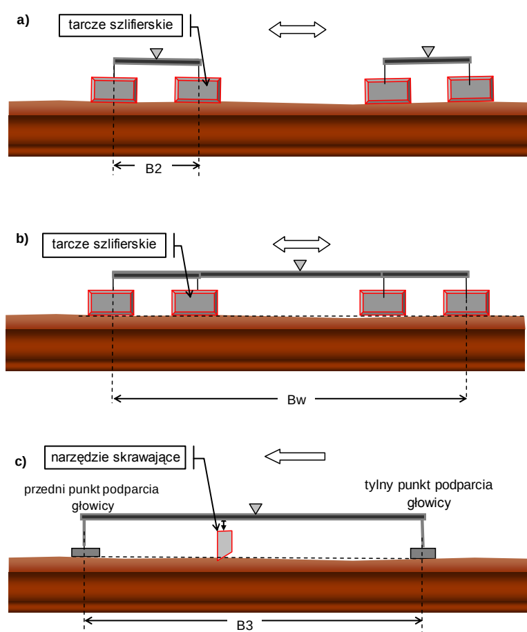
Rys. 11 Schemat ideowy baz odniesienia przy reprofilacji zmechanizowanej a) poprzez szlifowanie - dwupunktowa baza odniesienia przy usuwaniu fal krótkich b) poprzez szlifowanie - wielopunktowa baza odniesienia przy usuwaniu fal długich c) poprzez struganie lub frezowanie - 3-punktowa stała baza odniesienia
