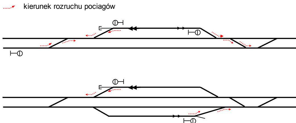
Rys. 5 Przykłady rozjazdów szczególnie narażonych na powstawanie wad 2223
