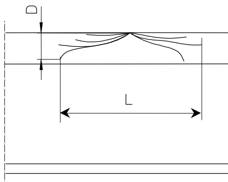
Rys. 10 Charakterystyczne parametry wad typu SQUAT
