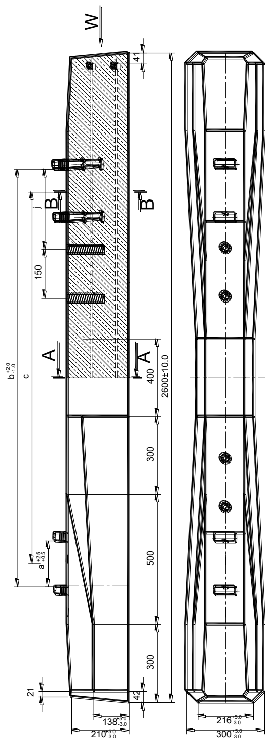
Podkład strunobetonowy PS-94M
