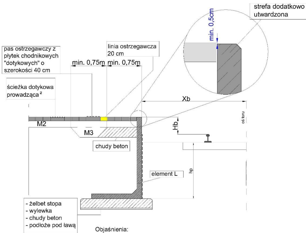
Rysunek nr 2 - System peronowy L
