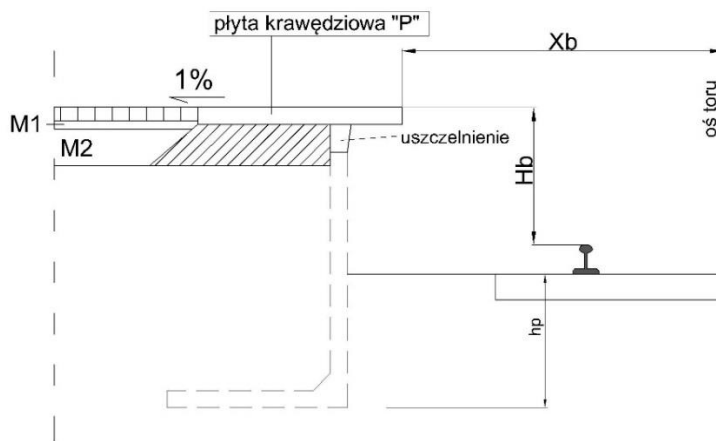
Rysunek nr 3 – System peronowy P
