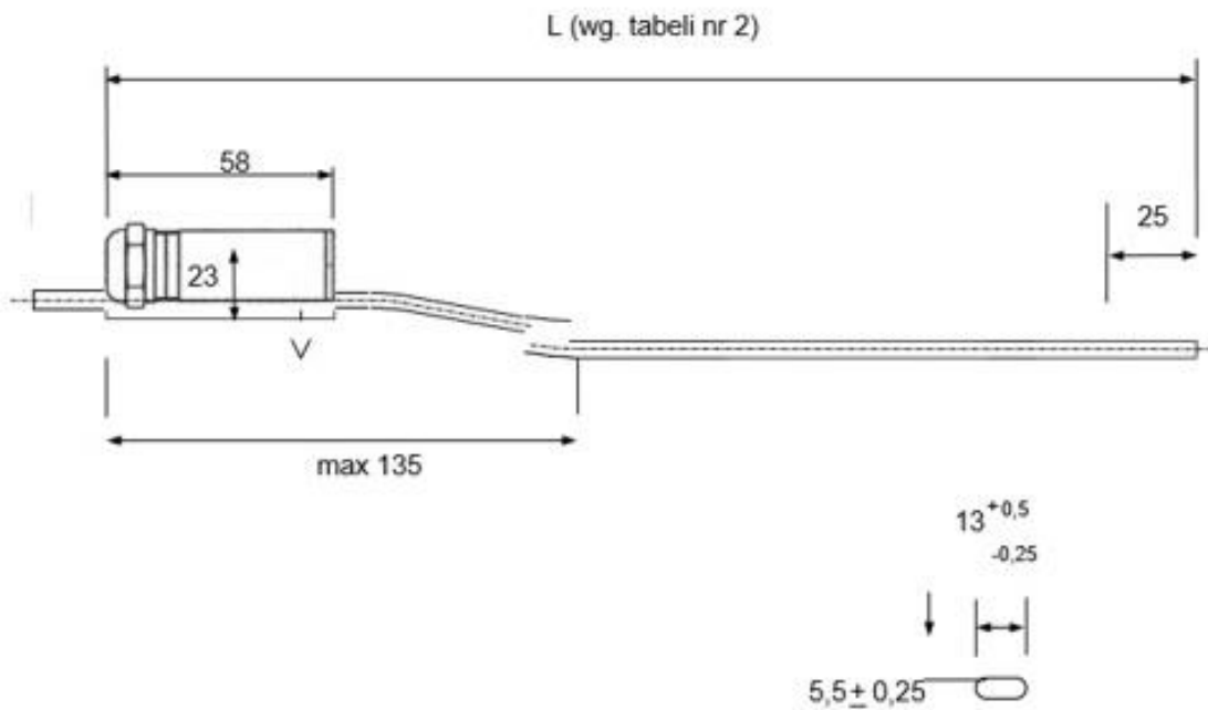
Rys 8. Grzejnik krzyżownicowy (do ogrzewania szyny skrzydłowej rozjazdu z ruchomym dziobem).
