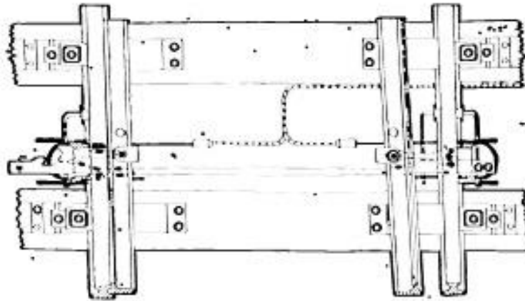
Rys. 1. Umieszczenie urządzenia do ogrzewania zamknięć nastawczych typu EGH -1.
