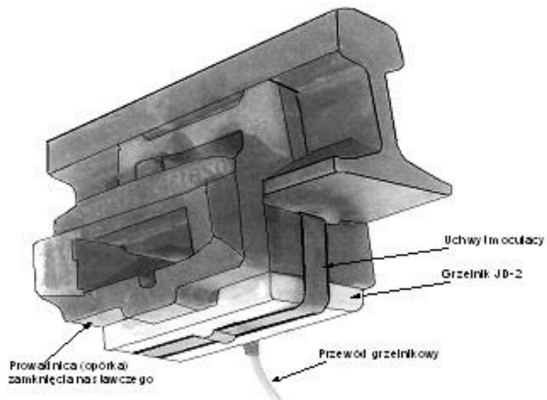
Rys. 6. Przykład mocowania grzejnika JD 2 pod zamknięciem nastawczym.
