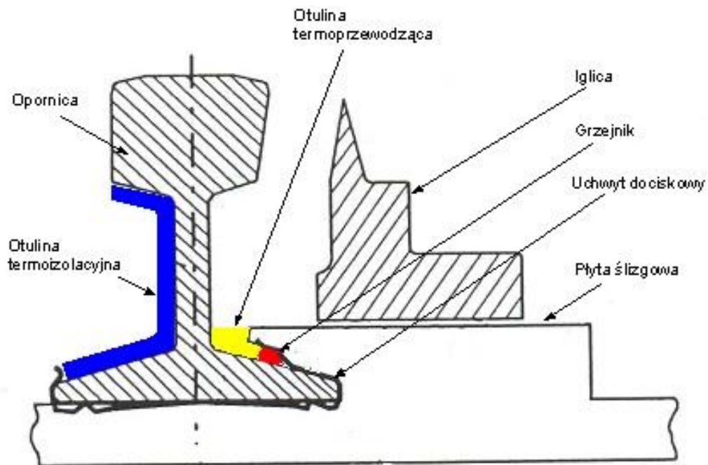
Rys 2. Sposób ułożenia otulin (termoizolacyjnej i termoprzewodzącej) oraz grzejnika w rozjeździe z mocowaniem opornic typu sprężystego z zastosowaniem uchwytów typu Df-2
