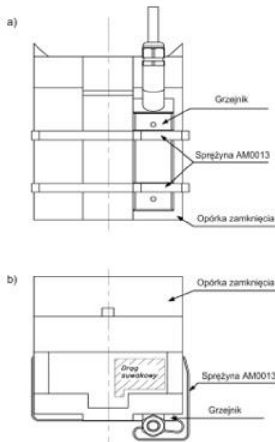
Rys. 7. Sposób mocowania grzejnika GZN – 01.
