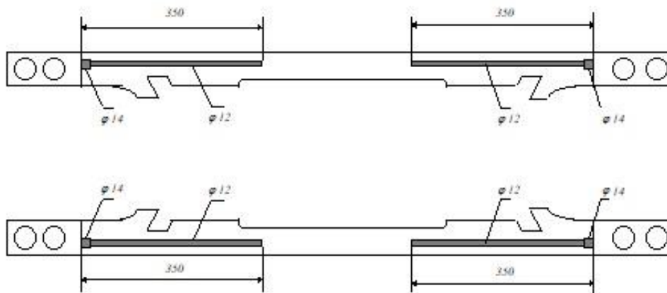
Rys. 5 Ogrzewanie zamknięcia nastawczego typu K. Lokalizacja otworów na grzejniki EG-50 w drążku suwakowym. U góry suwak lewy, u dołu suwak prawy.
