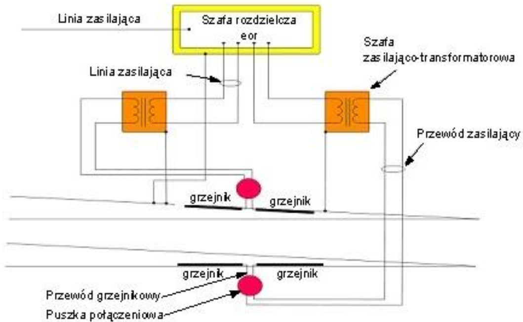
Rys. 1. Schemat ideowy urządzeń eor (zasilanie grzejników opornicowych).
