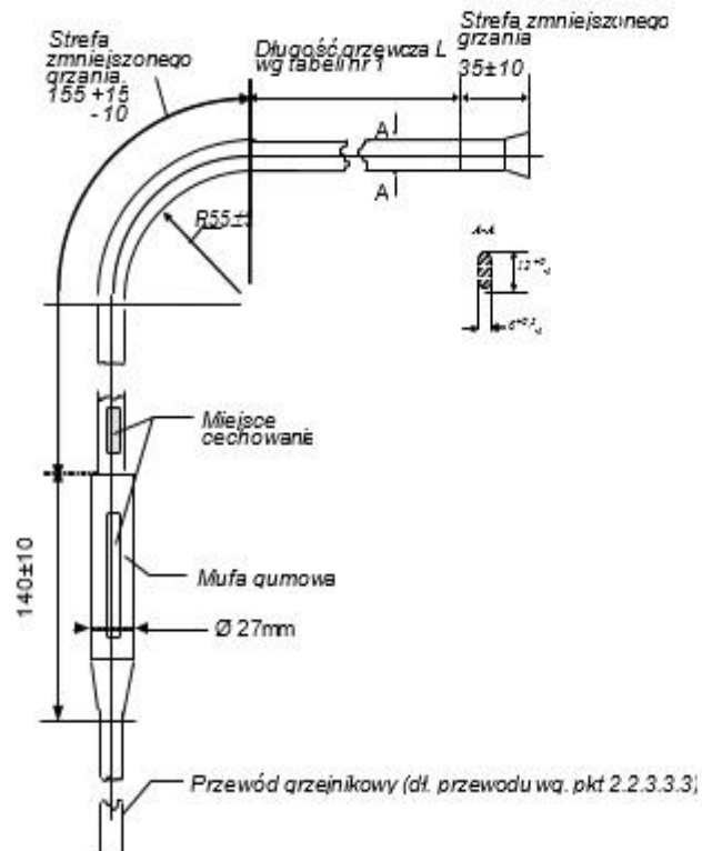
Rys. 1. Grzejnik opornicowy z długim ramieniem i mufą gumową.
