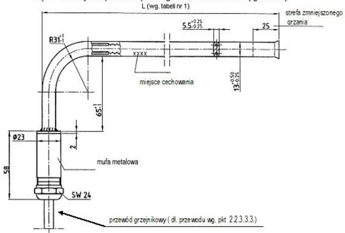
Rys. 2. Grzejnik opornicowy z krótkim ramieniem i mufą metalową.
