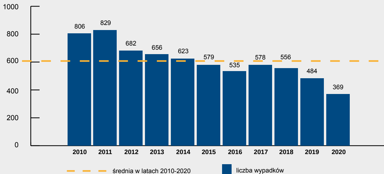
Porównanie liczby wypadków, do których doszło w latach 2010-2020 na liniach kolejowych zarządzanych przez PKP Polskie Linie Kolejowe S.A.
