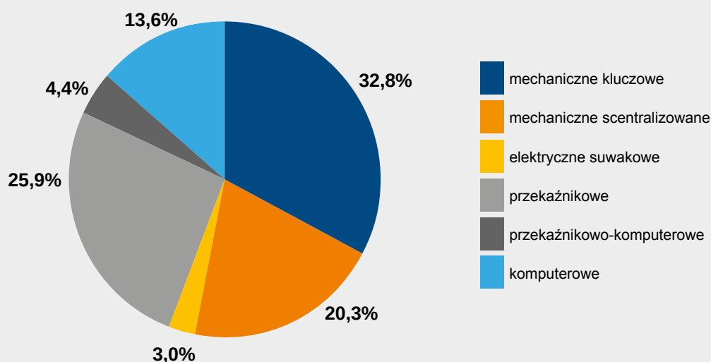
Okręgi nastawcze w poszczególnych rodzajach stacyjnych urządzeń srk
