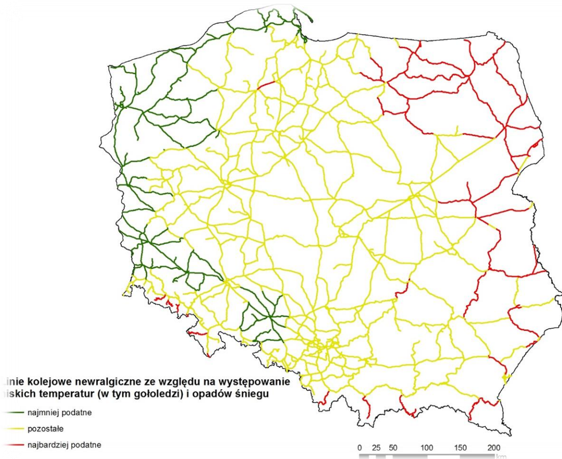
Rysunek 3 Mapa najbardziej i najmniej podatnych linii kolejowych na niskie temperatury (w tym gołoledź) i opady śniegu, z uwzględnieniem prognozowanych zmian według scenariusza RCP 8.5 Źródło: opracowanie własne
