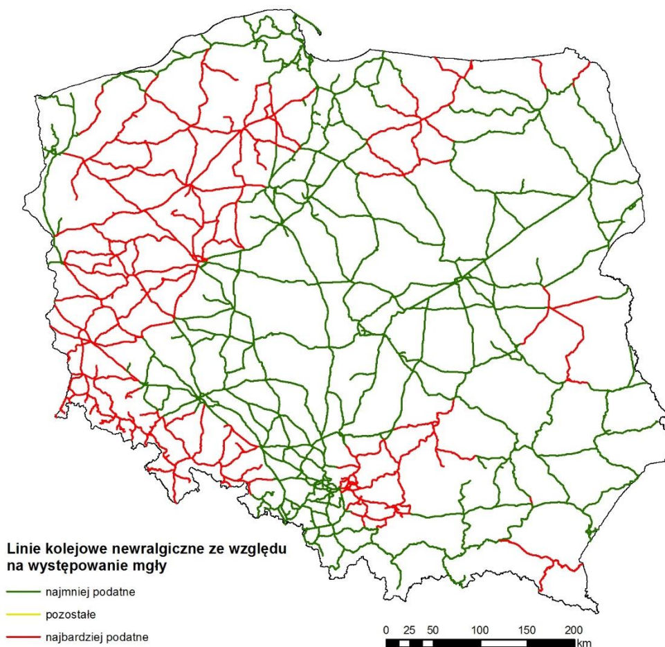
Rysunek 8 Mapa najbardziej i najmniej podatnych linii kolejowych na występowanie mgły, z uwzględnieniem prognozowanych zmian według scenariusza RCP 8.5 Źródło: opracowanie własne
