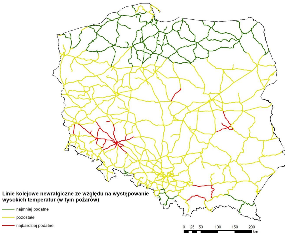
Rysunek 4 Mapa najbardziej i najmniej podatnych linii kolejowych na wysokie temperatury (w tym pożary), z uwzględnieniem prognozowanych zmian według scenariusza RCP 8.5
