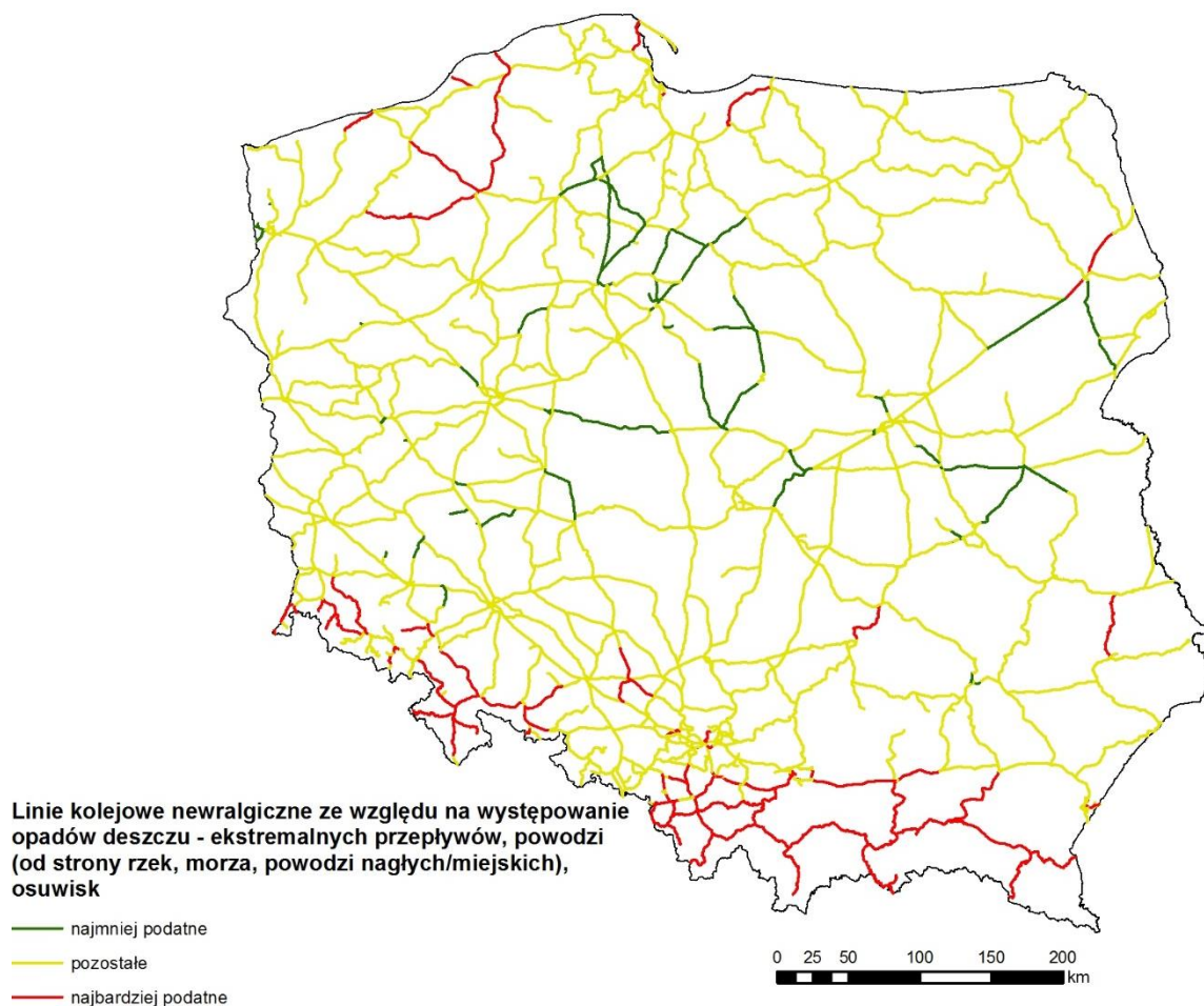
Rysunek 7 Mapa najbardziej i najmniej podatnych linii kolejowych na występowanie opadów deszczu – ekstremalnych przepływów, powodzi (od strony rzek, morza, powodzi nagłych/miejskich), osuwisk, z uwzględnieniem prognozowanych zmian według scenariusza RCP 8.5
