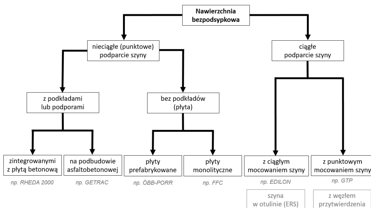
Rys. 1 Podział konstrukcji nawierzchni bezpodсыpkowej
